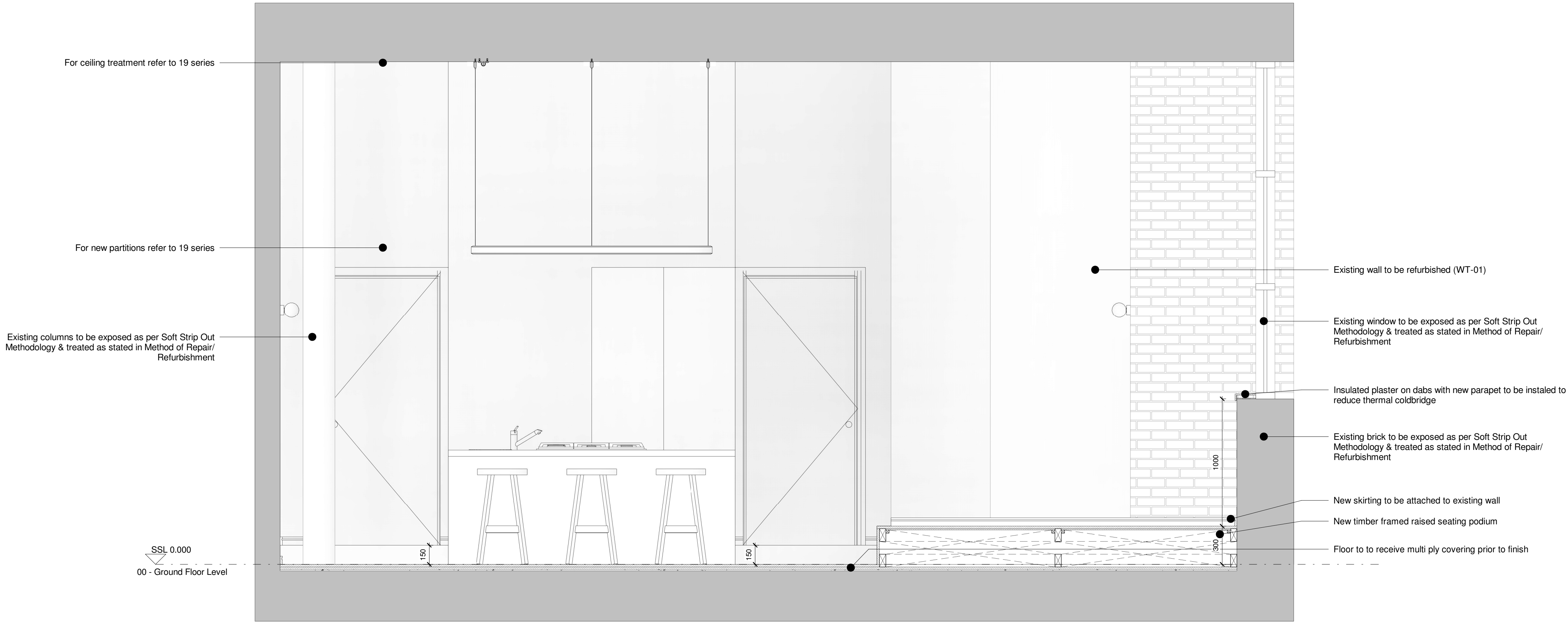
Section 1 Scale: 1 : 20
