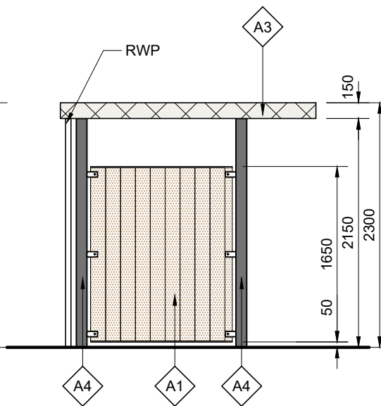
L.H. SIDE ELEVATION
