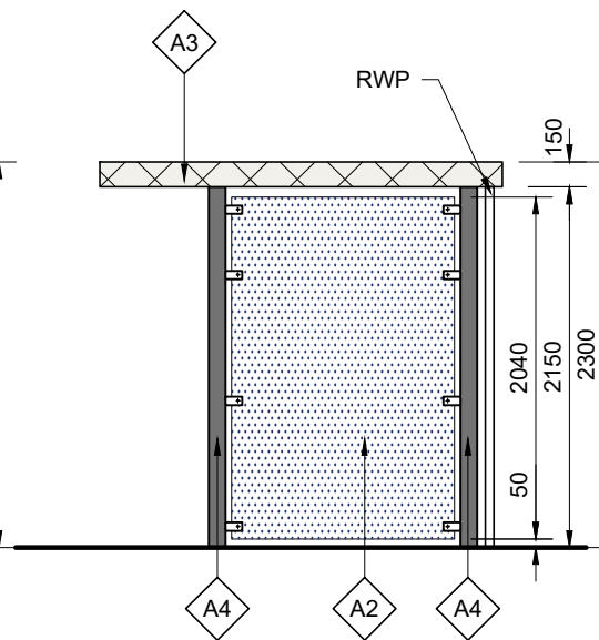
R.H. SIDE ELEVATION
