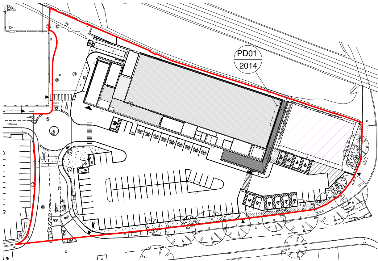
KEY PLAN 1 : 1000
