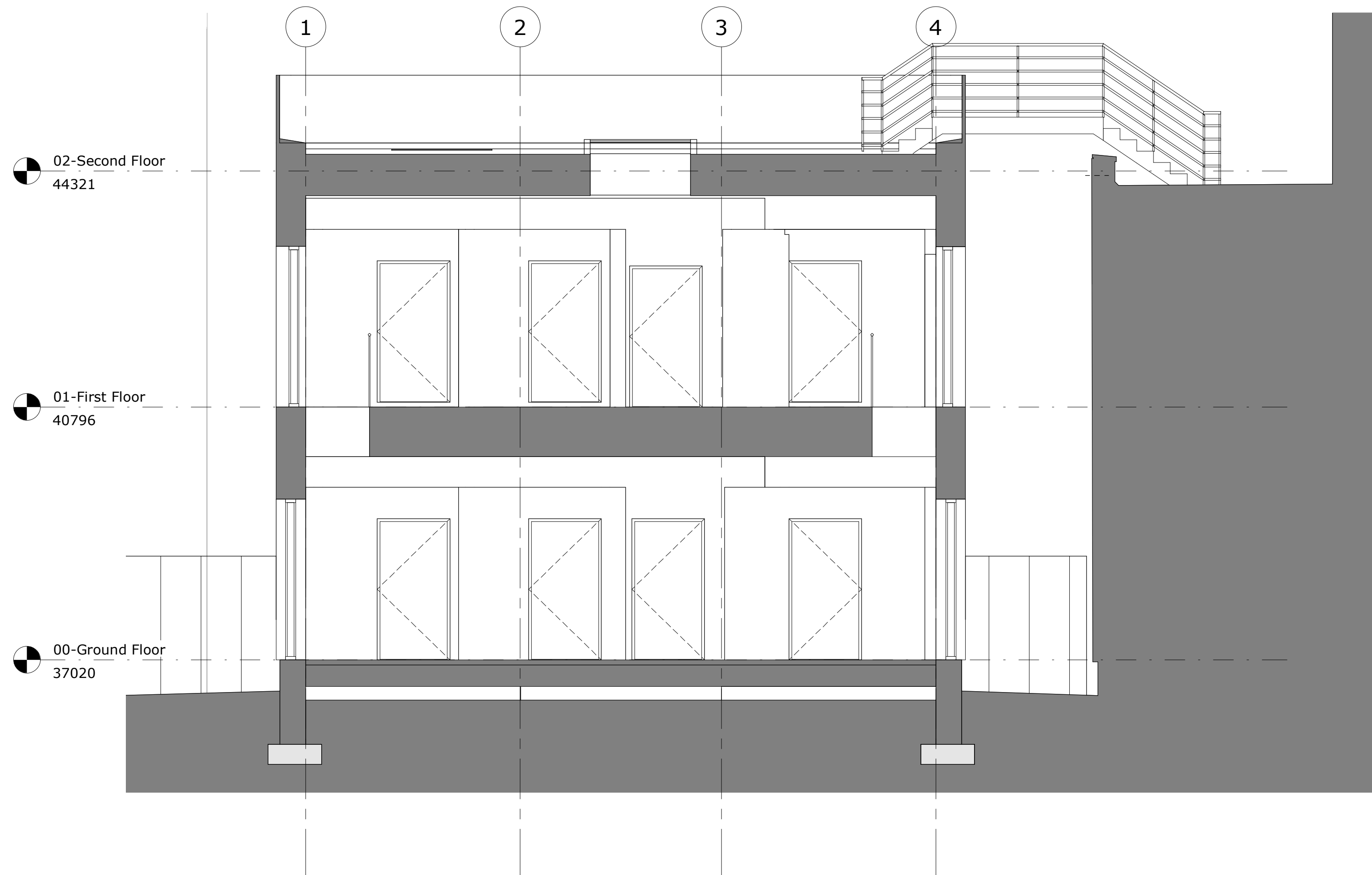
B Section B-B SCALE: 1 : 50
