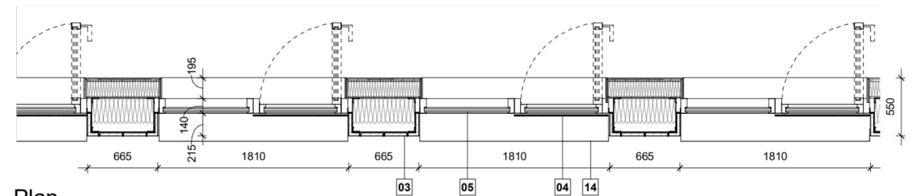
Plan 1 : 50
