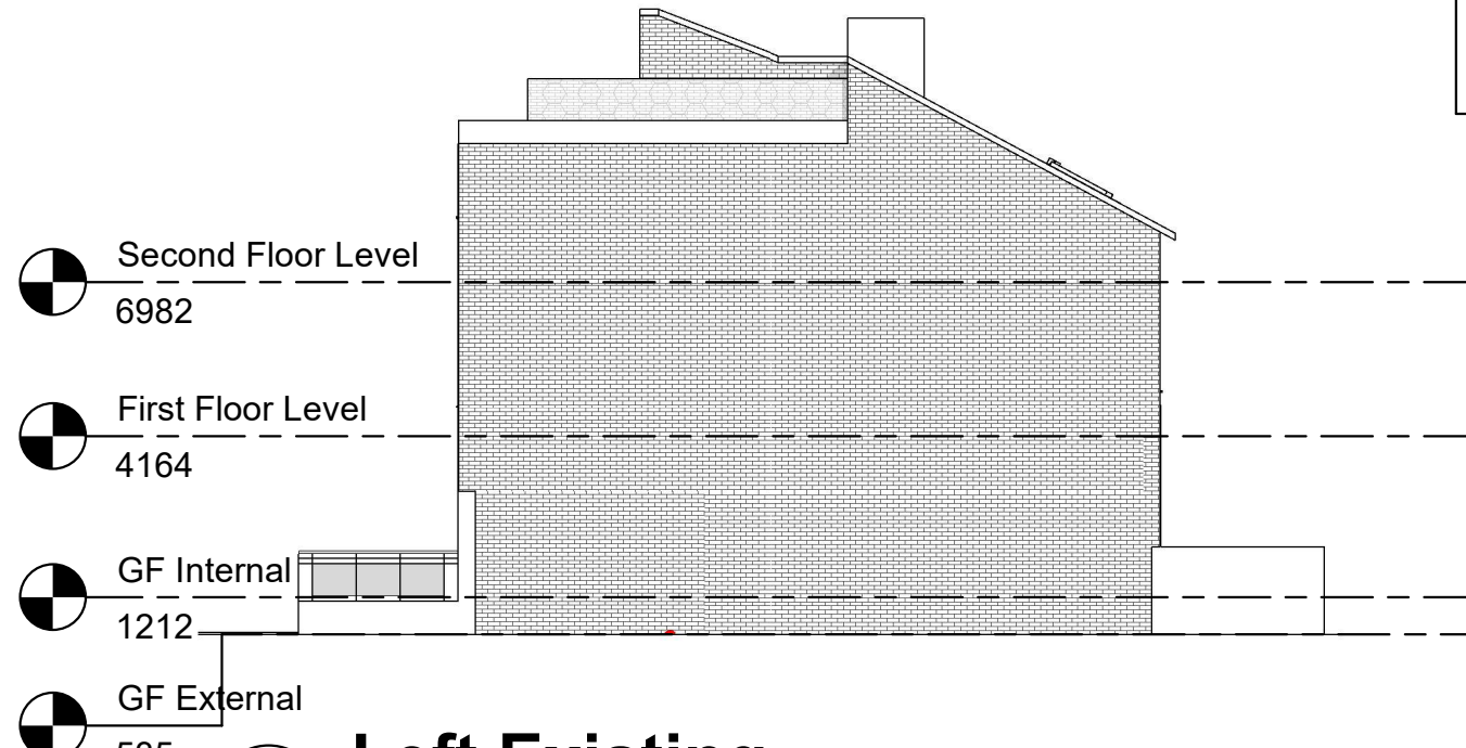
2 Left Existing 1 : 150
