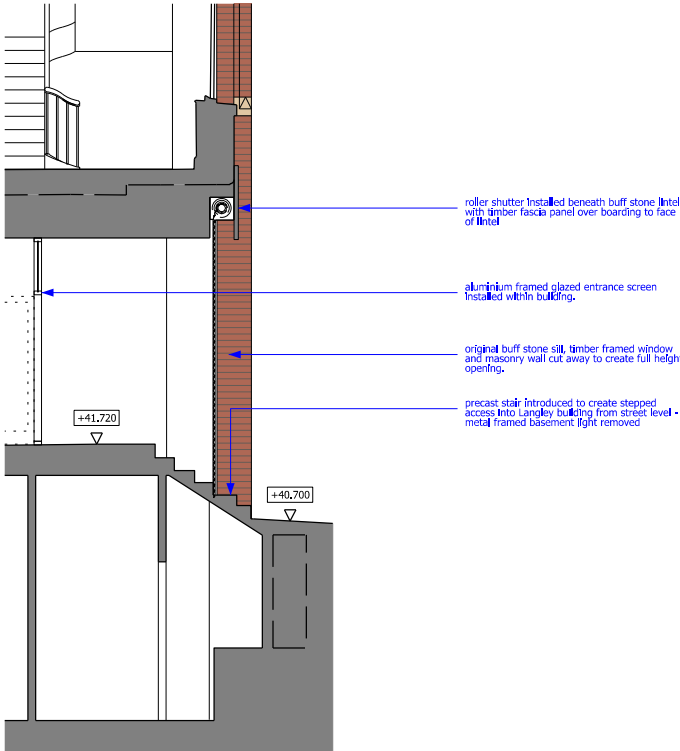
Existing Section A-A 1:50
