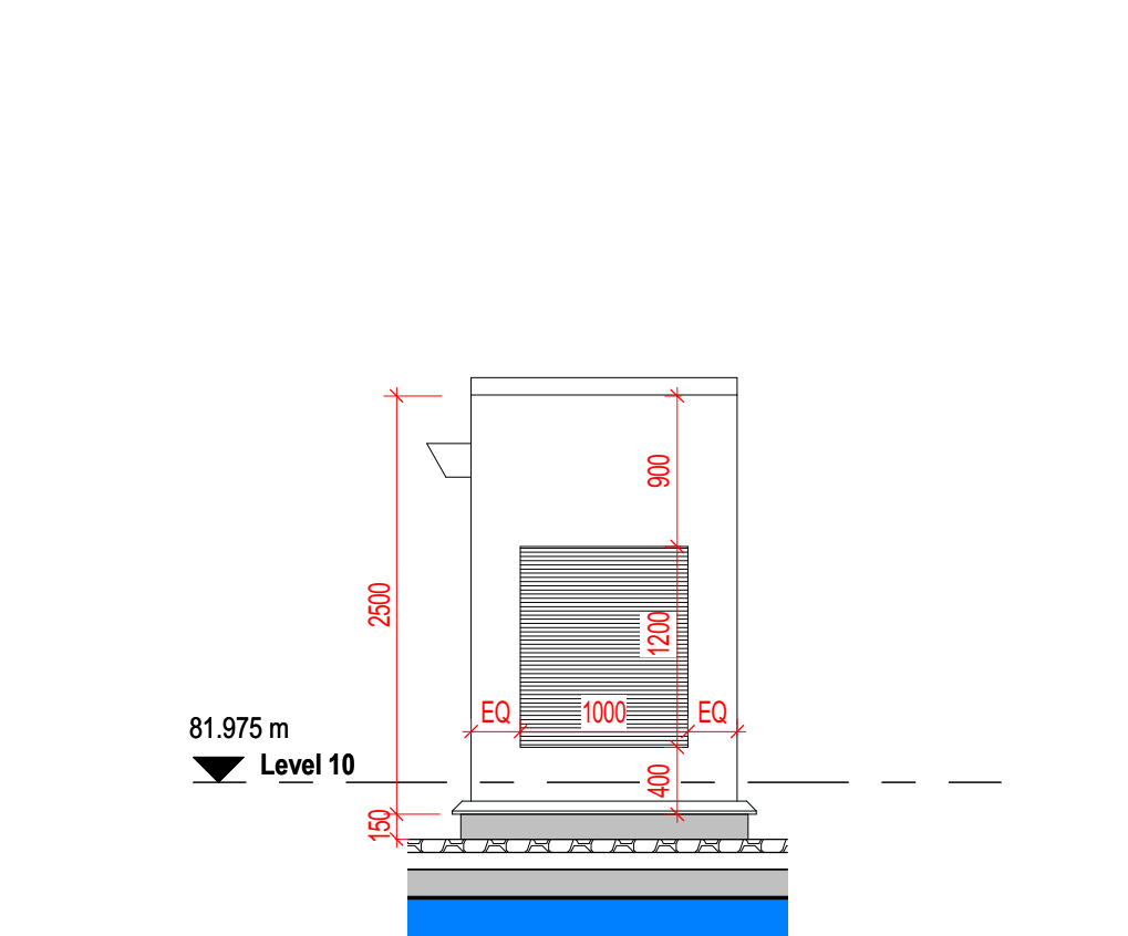
SE2 - Elevation 4
