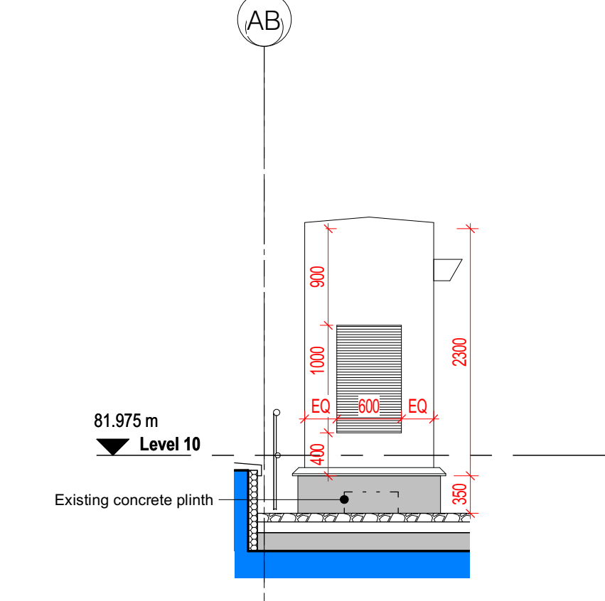
SE3 - Elevation 3
