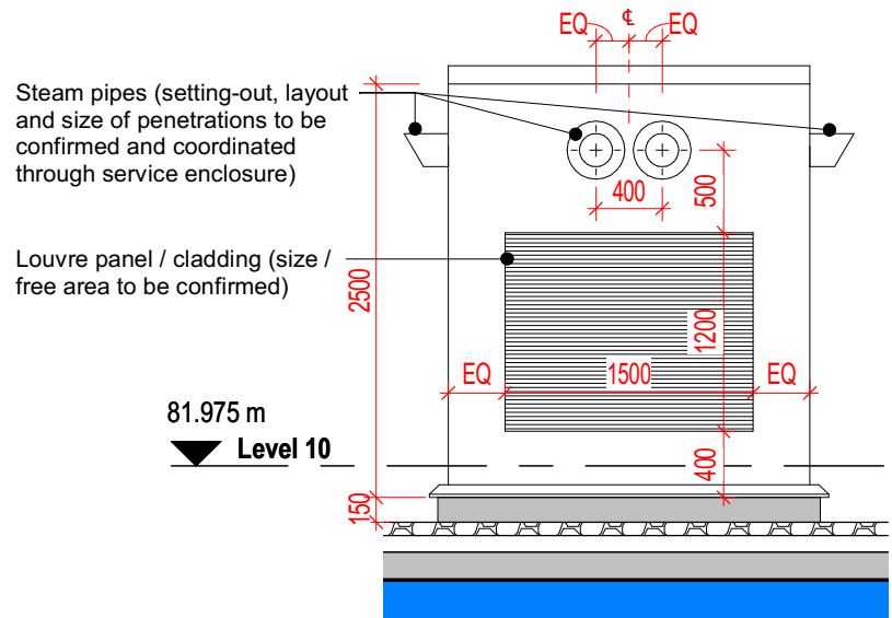
SE1 - Elevation 2
