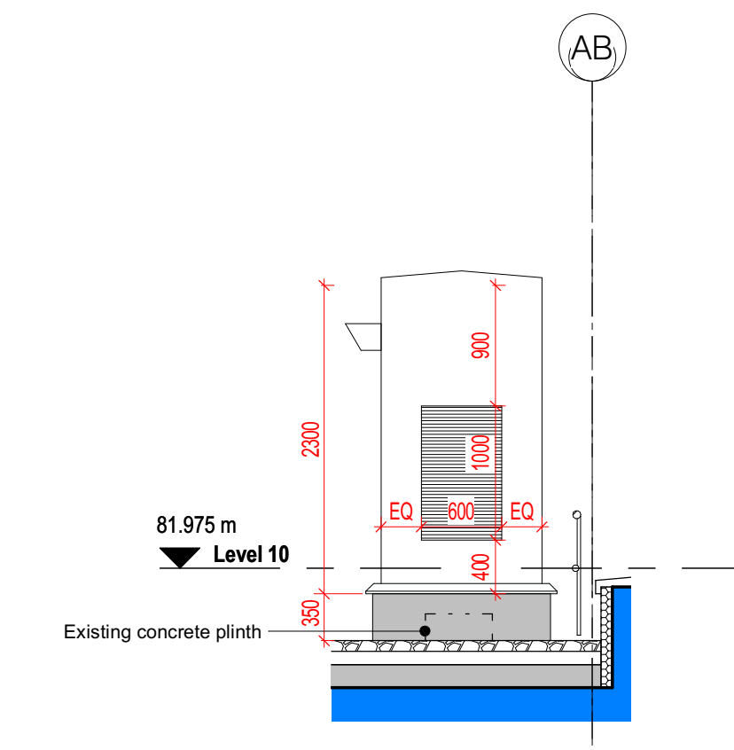
SE3 - Elevation 1
