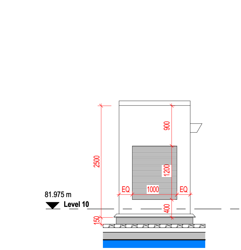
SE2 - Elevation 2
