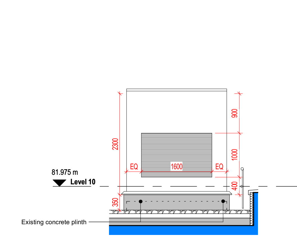
SE3 - Elevation 4
