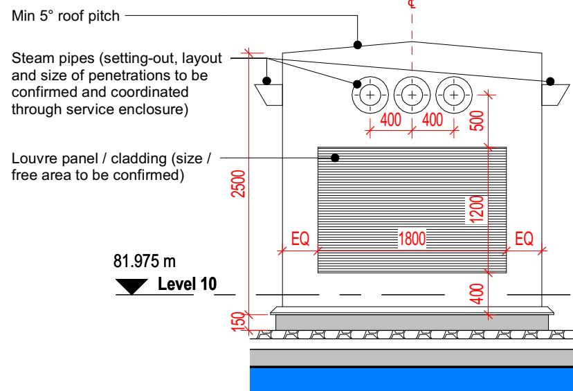
SE1 - Elevation 1
