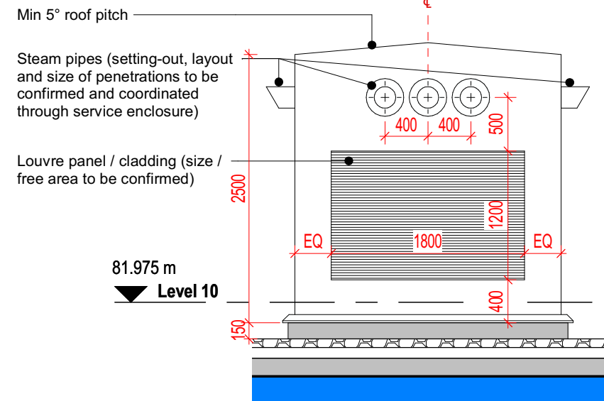
SE1 - Elevation 3
