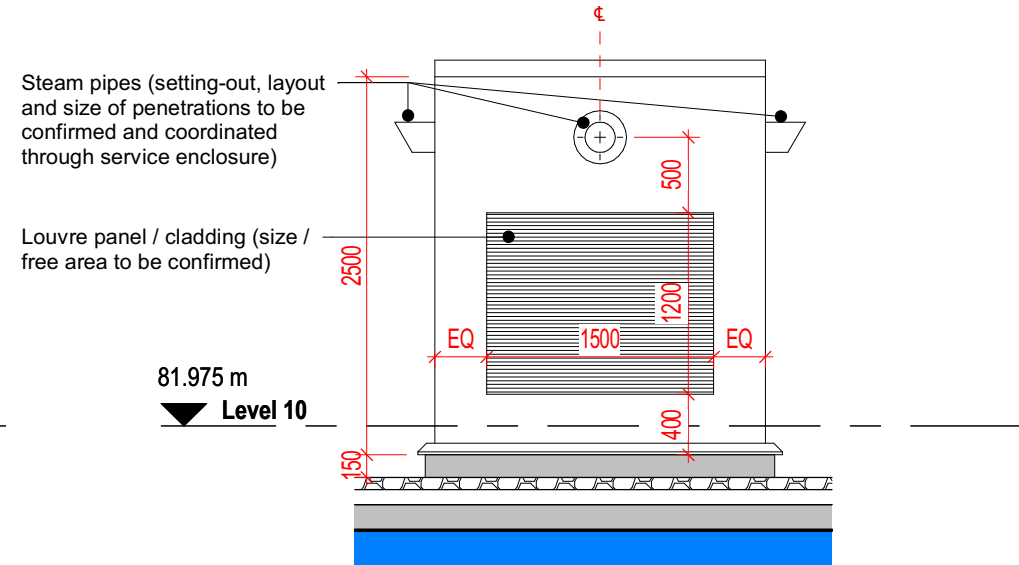
SE1 - Elevation 4
