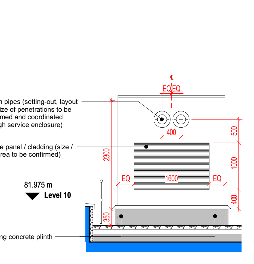
SE3 - Elevation 2
