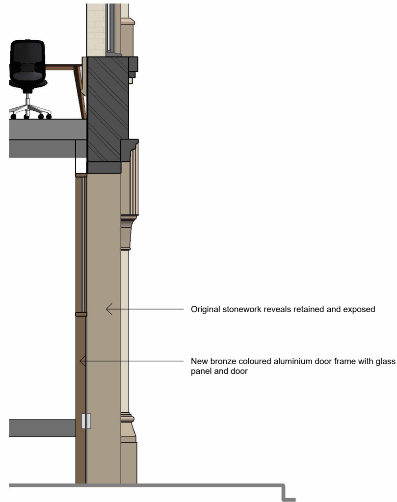
3 Section 1 : 50
