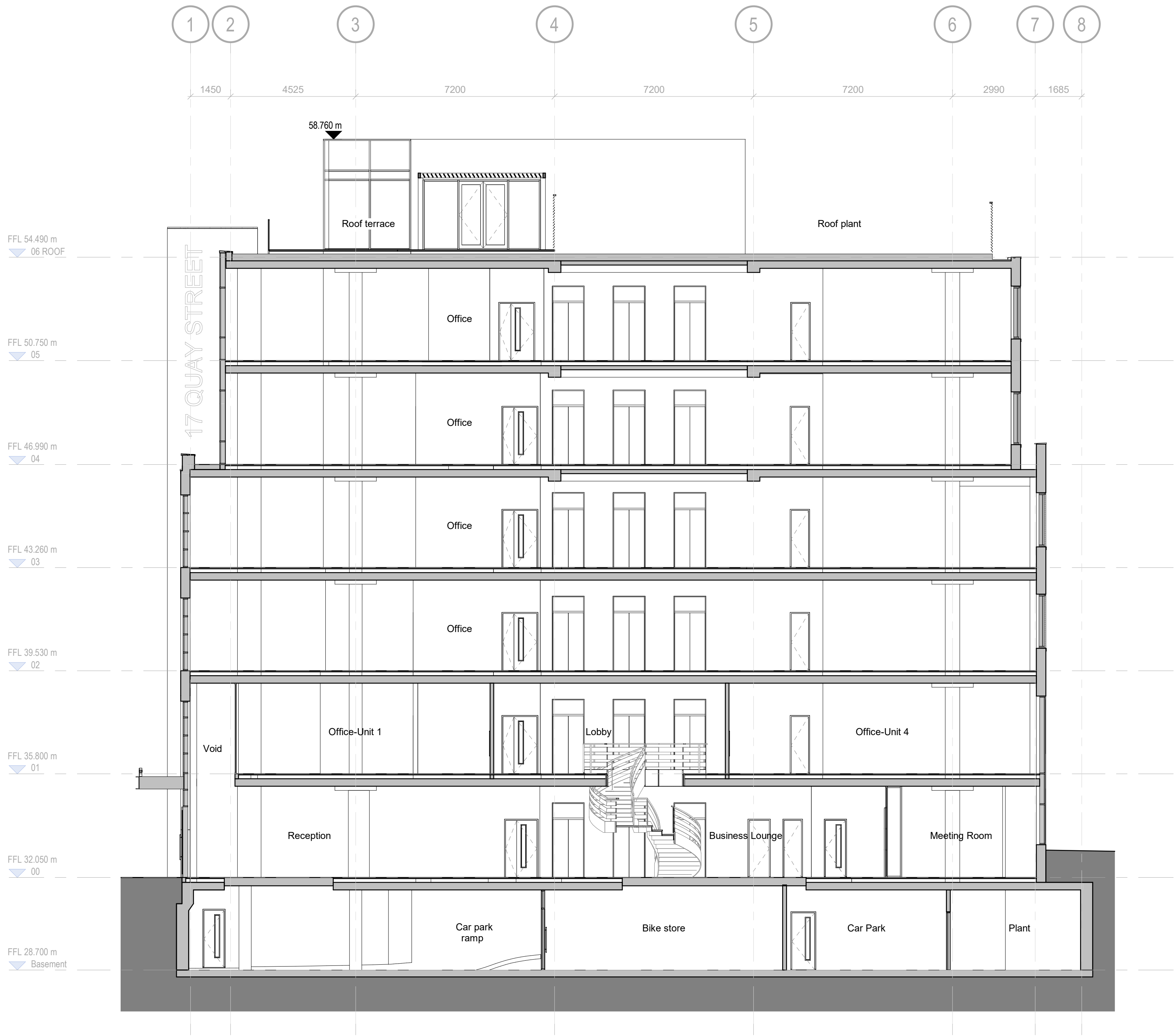
GA Section B-B 1 : 100
