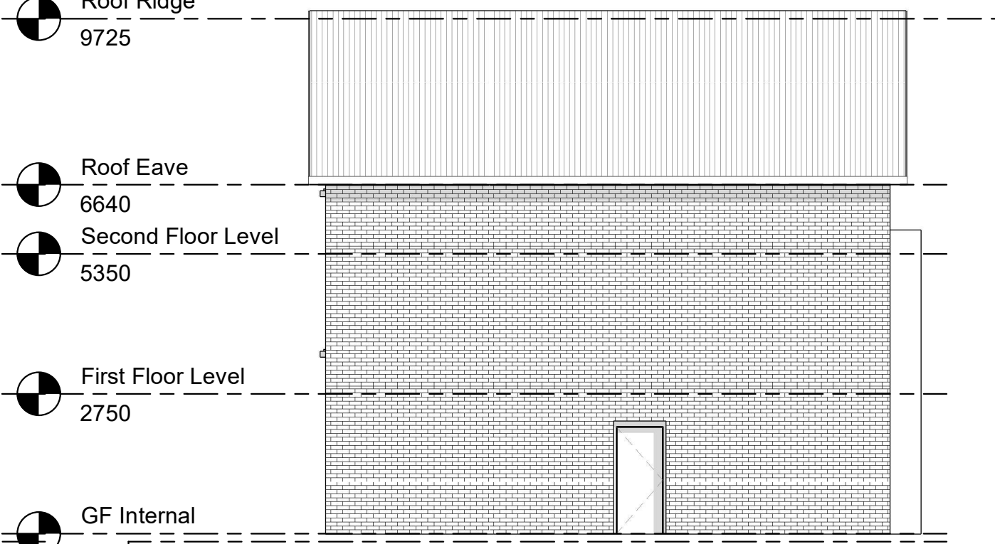
4 Left Existing 1 : 100
