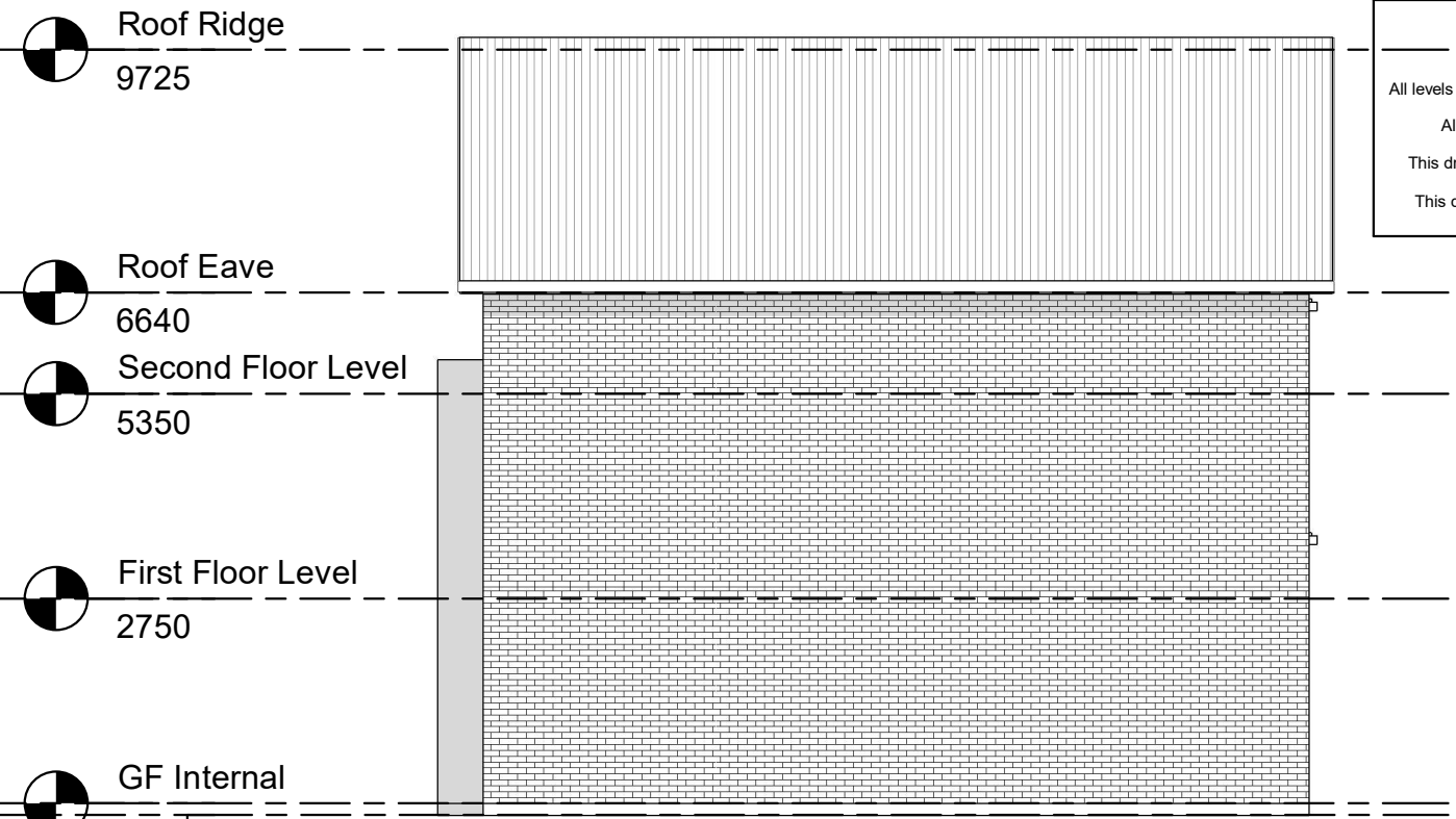
2 Right Existing 1 : 100
