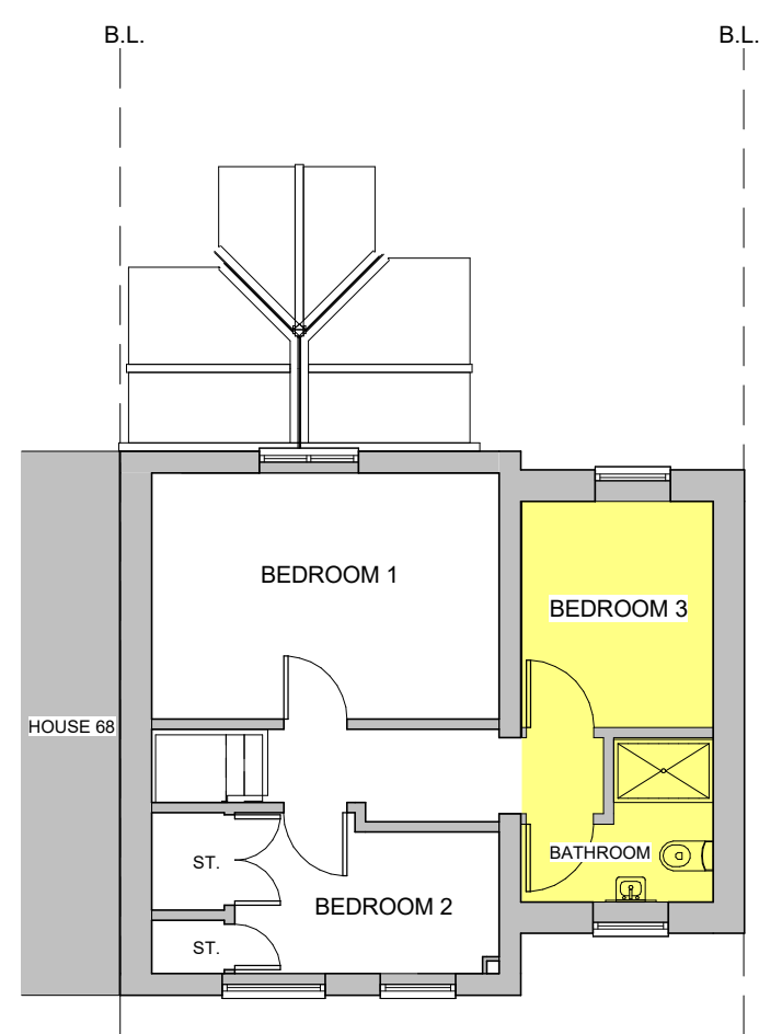
7 1/F 1 : 100
