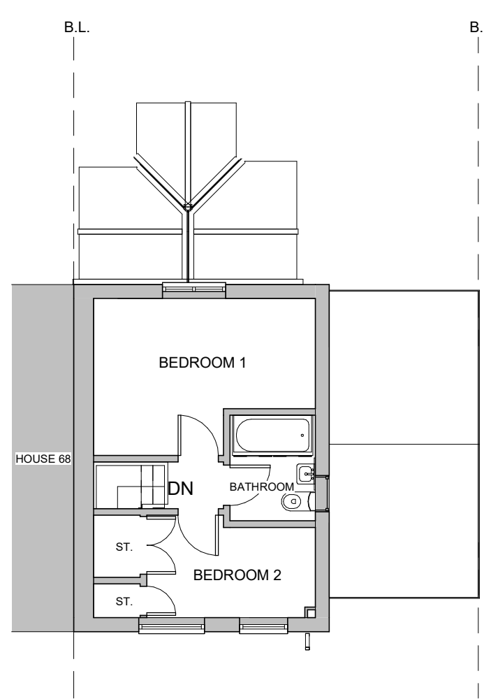
5 Existing 1/F 1 : 100
