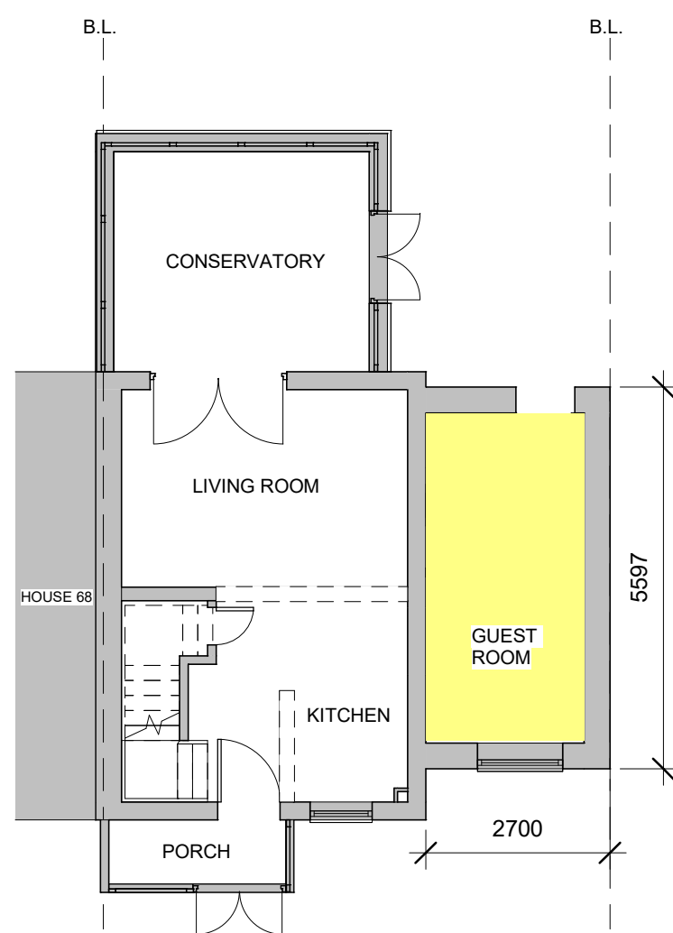
6 G/F 1 : 100
