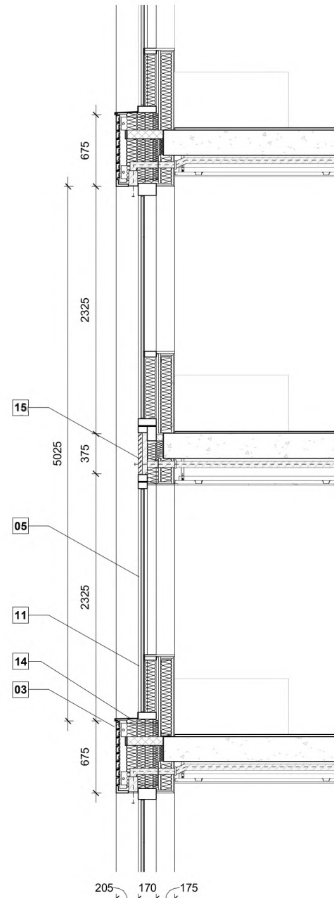
Section - Window 1 : 50
