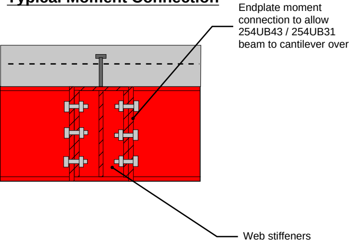
Section 2 - 0200
