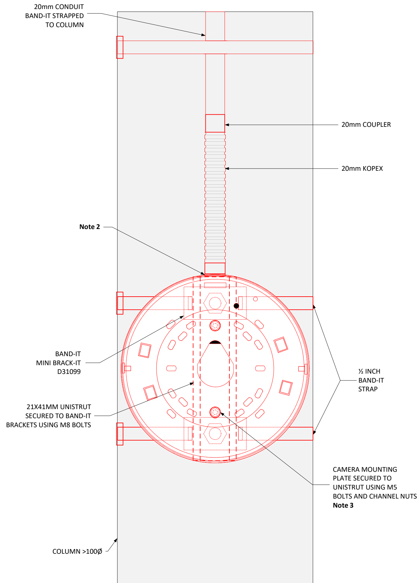
FRONT ELEVATIUN
