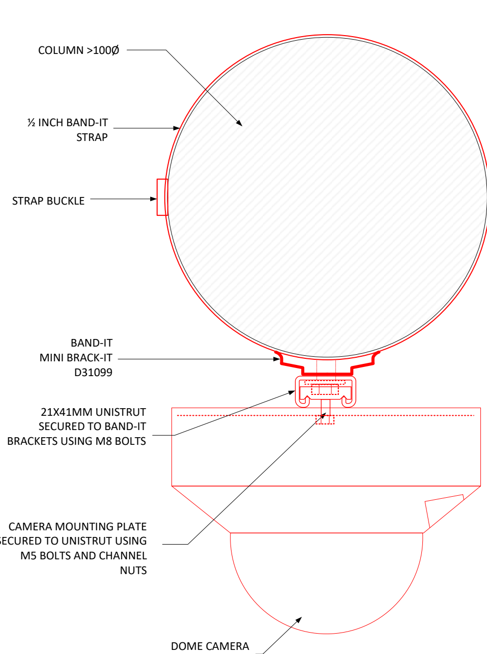
TOP ELEVATIUN
