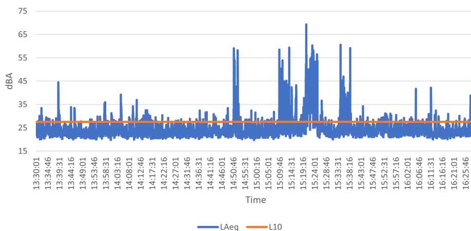
MP5 - LAeq & LA10 3Hr
