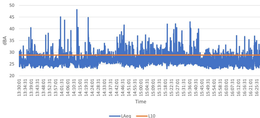
MP6 - LAeq & LA10 3Hr
