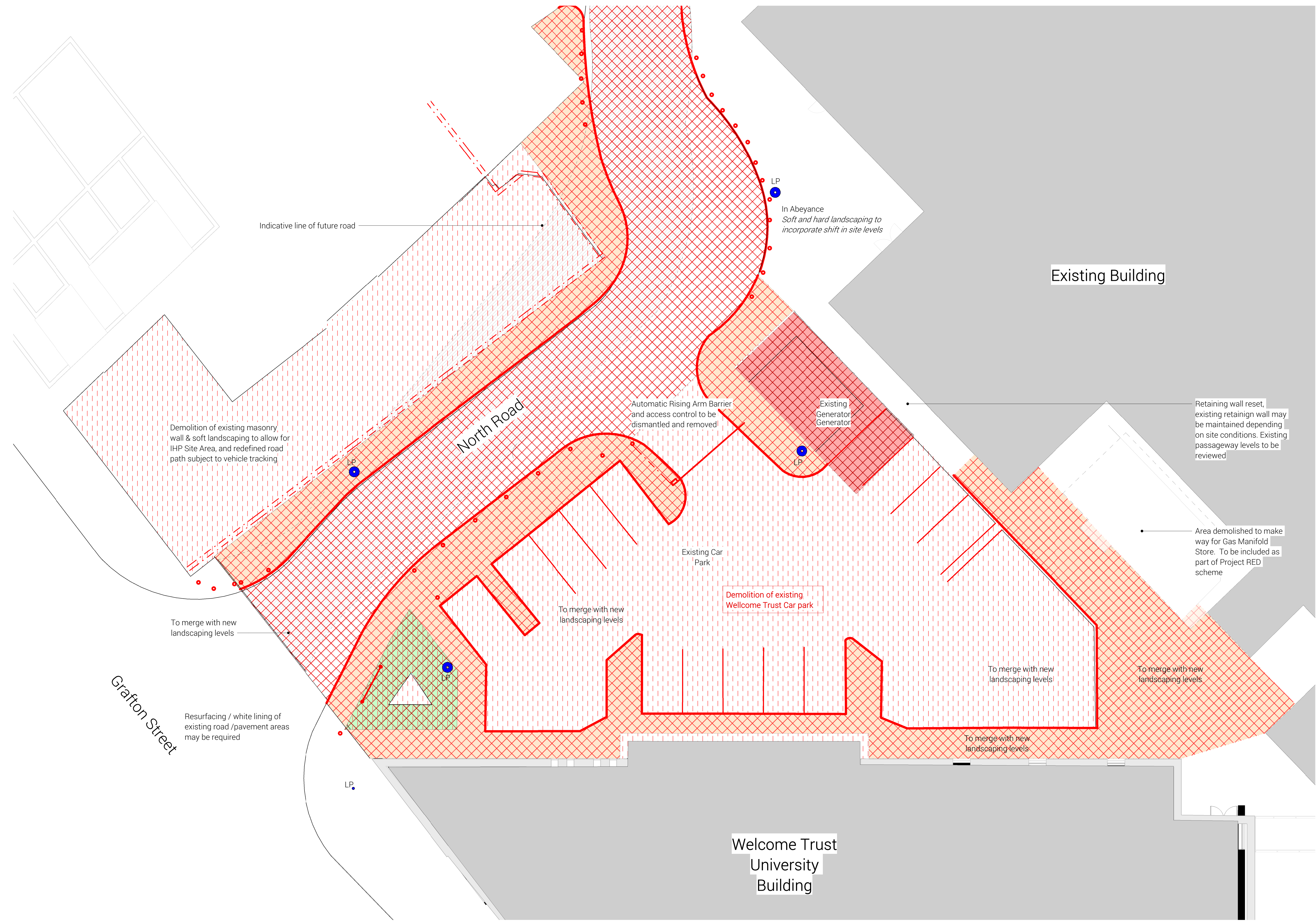
1 Demolition Plan 1 : 100
