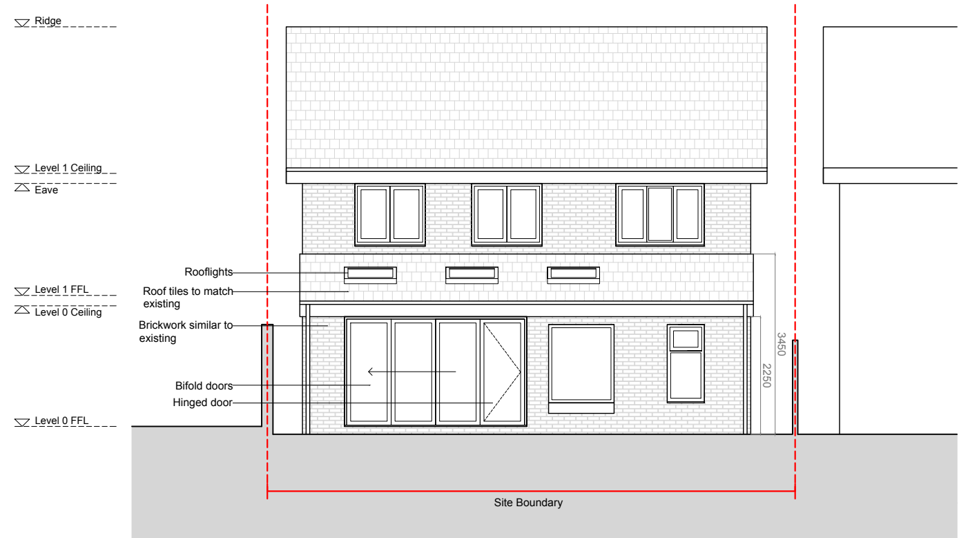
Elevation BB
