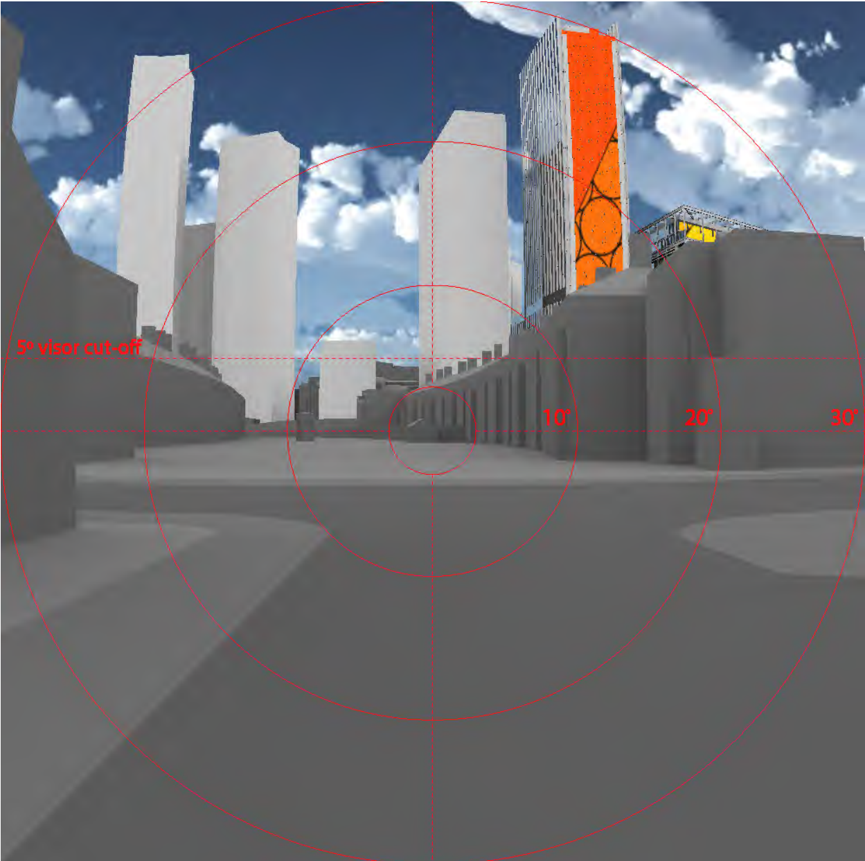
Fig. 141: Solar reflections
