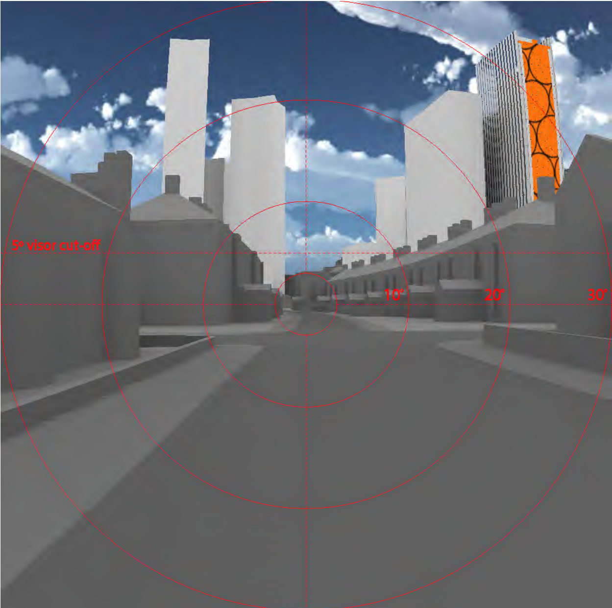
Fig. 146: Solar reflections
