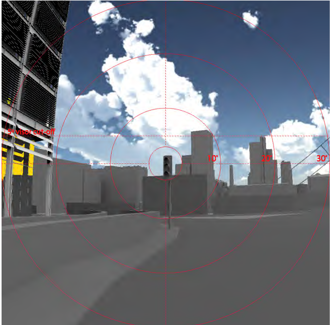
Fig. 137: Solar reflections
