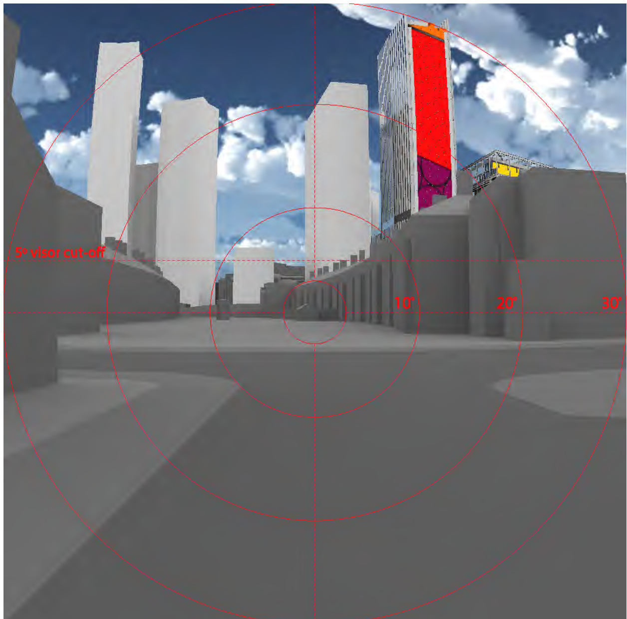
Fig. 142: Solar reflections
