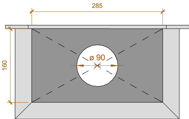
Plan 1:5
