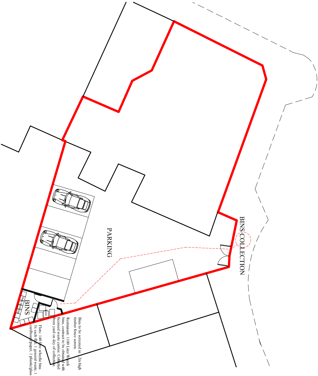
SITE PLAN 1:250
