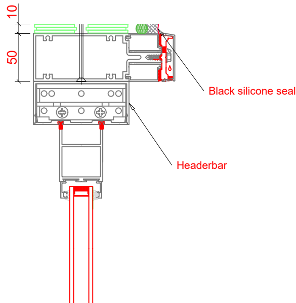
02 Door Head Detail - A Scale 1:4
