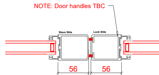
02 Door Meeting stiles Detail - J Scale 1:4
