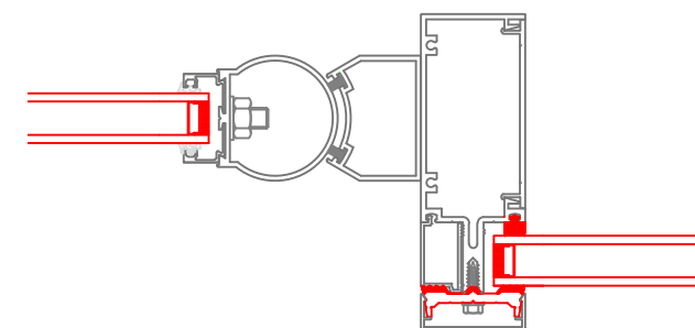
02 R/H Door Mullion Detail - K Scale 1:4
