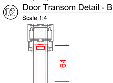
02 Door Transom Detail - B Scale 1:4
