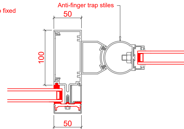
02 L/H Door Mullion Detail - H Scale 1:4
