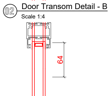
02 Door Transom Detail - B Scale 1:4
