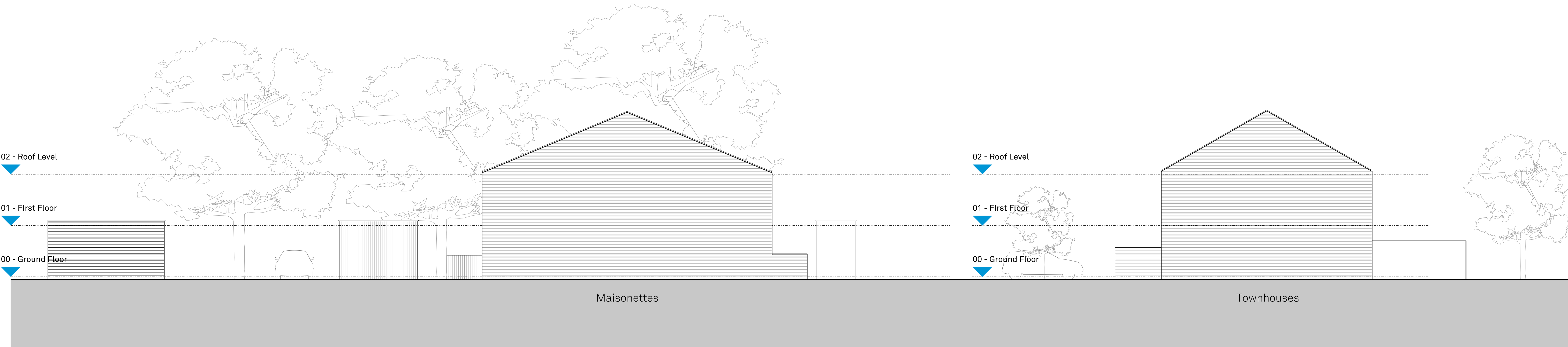
Site Elevation - 1:100
