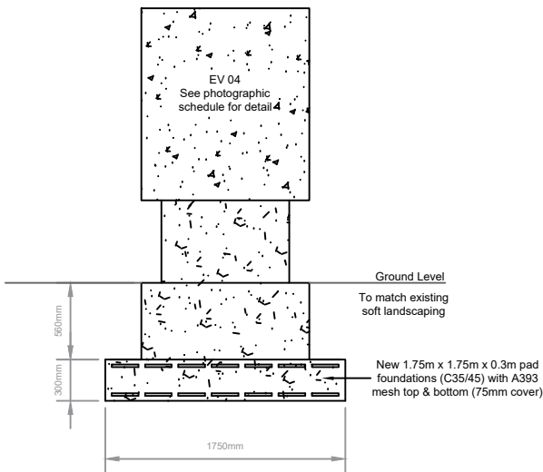
Elevation 04
