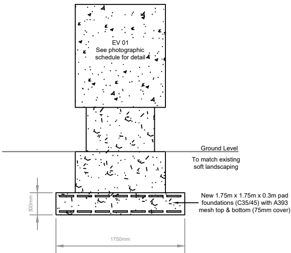
Elevation 01
