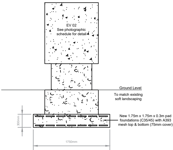
Elevation 02
