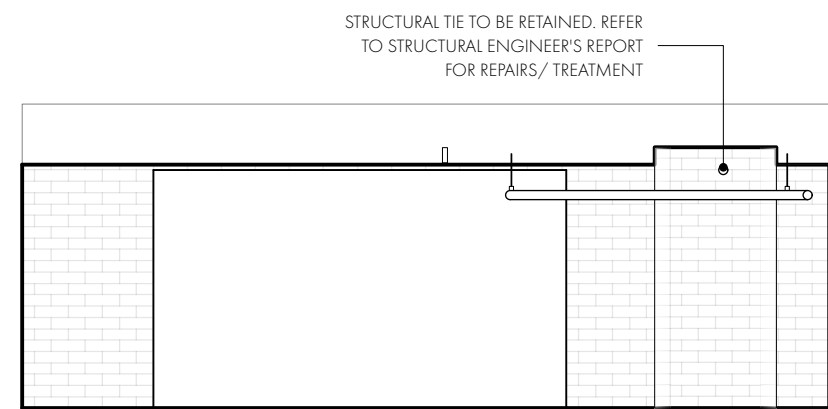
ELEVATION A
