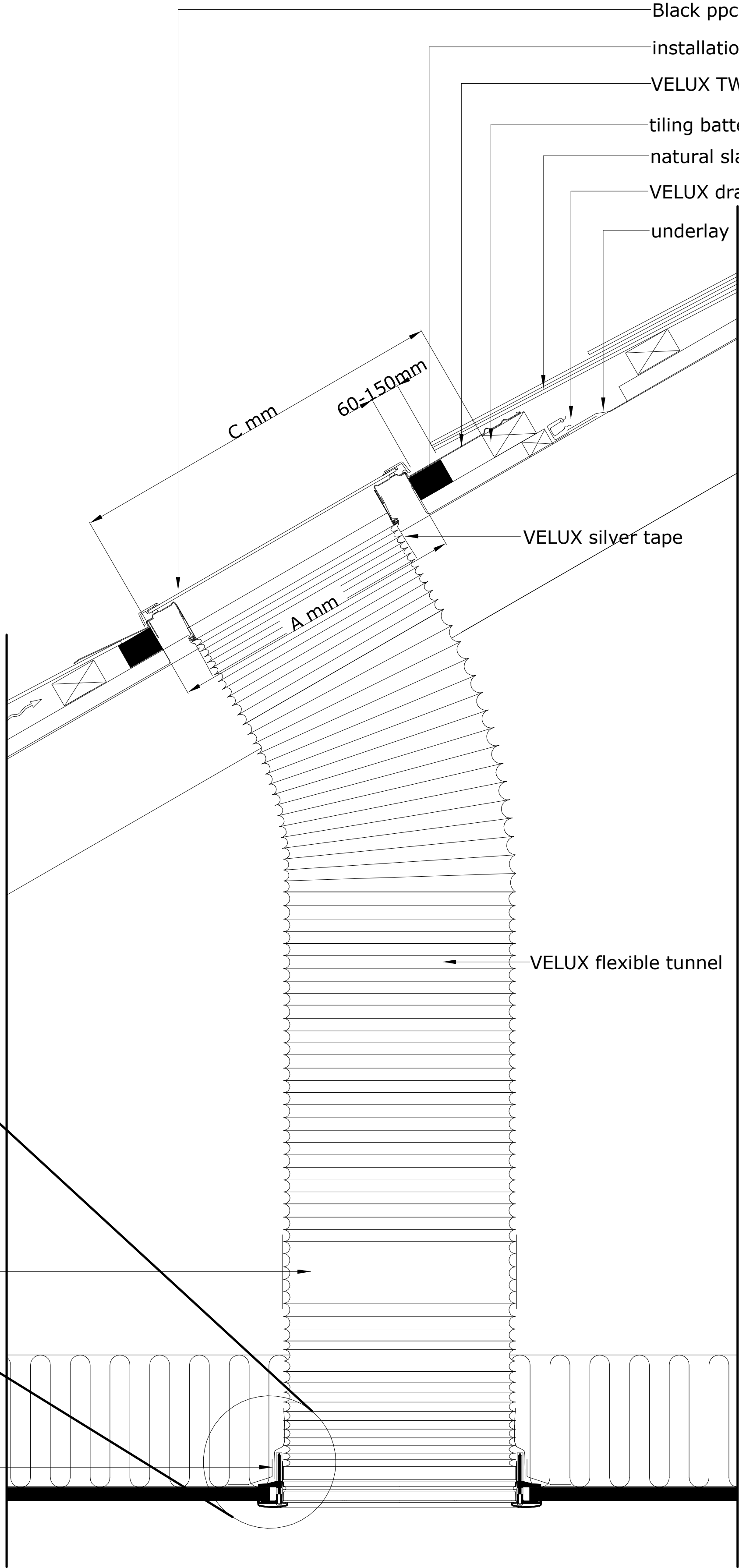
SECTION A-A
