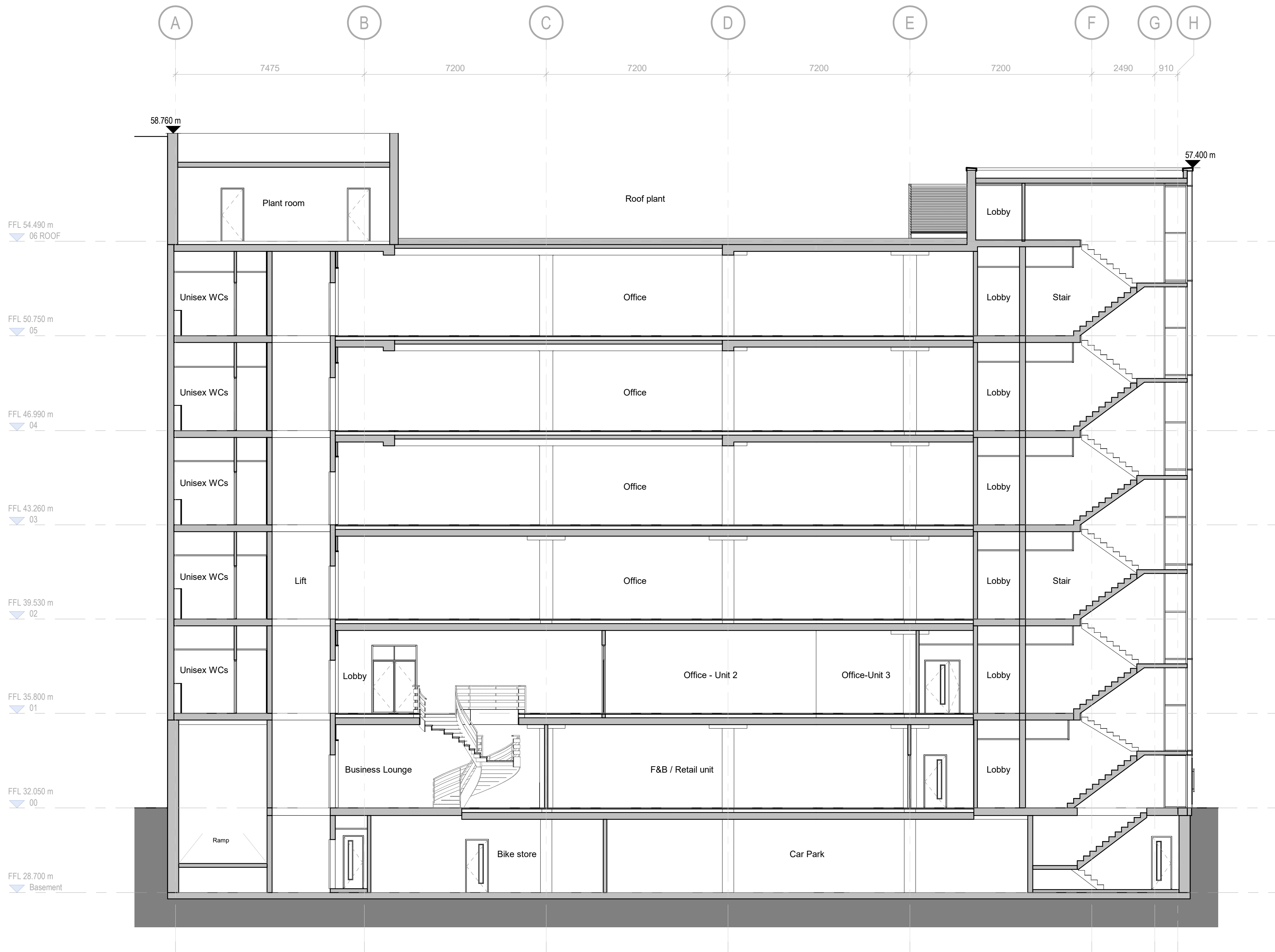
GA Section A-A 1 : 100
