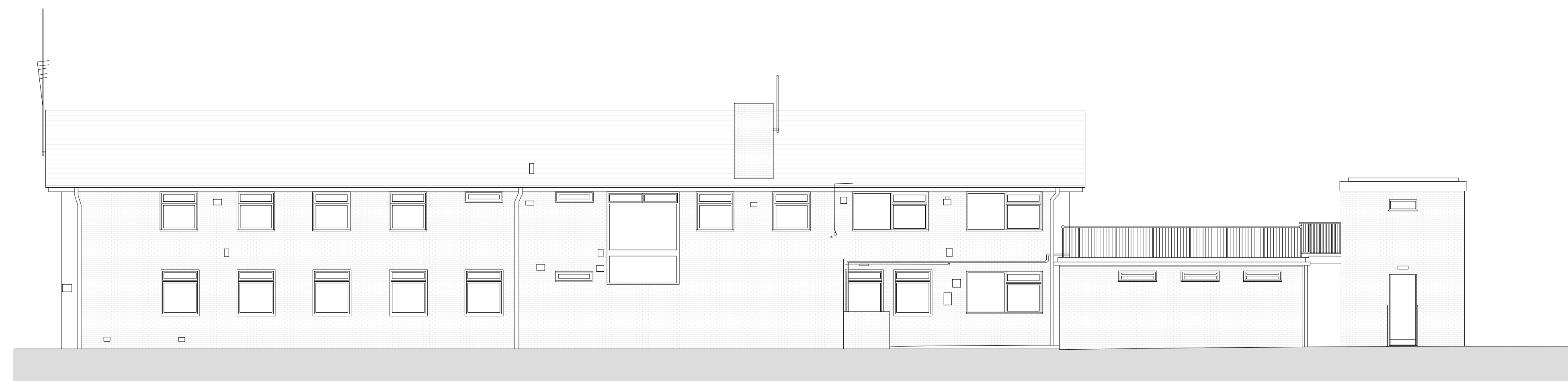
Elevation 4
