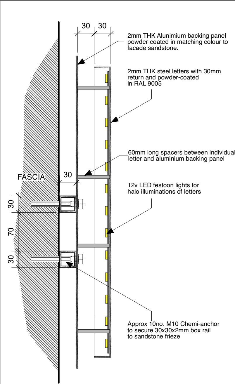
SECTION A-A - 1:4
