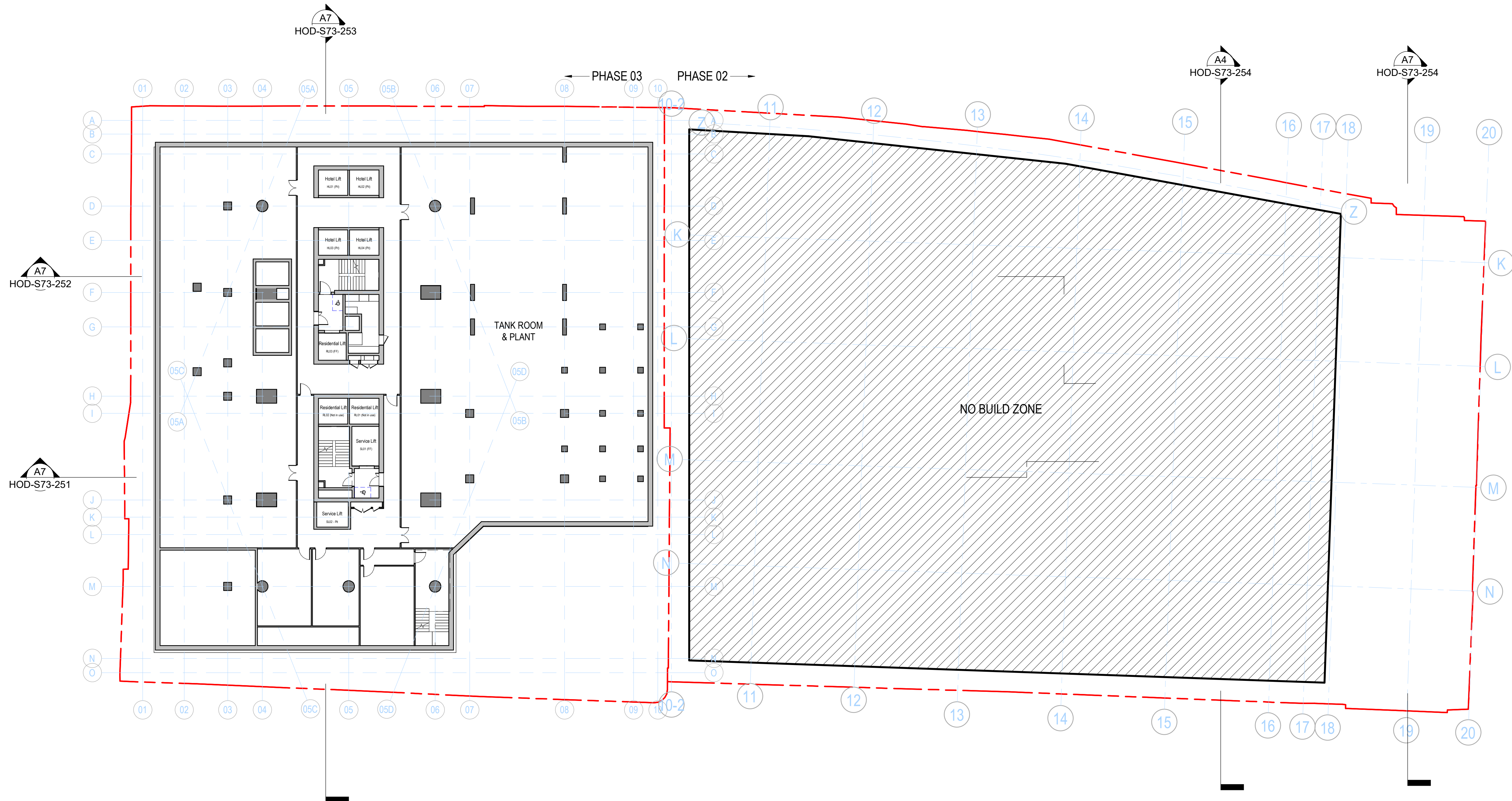
A7 LEVEL B3 PLAN 1 : 200
