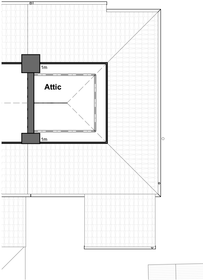
1 RF-Roof 1:100
