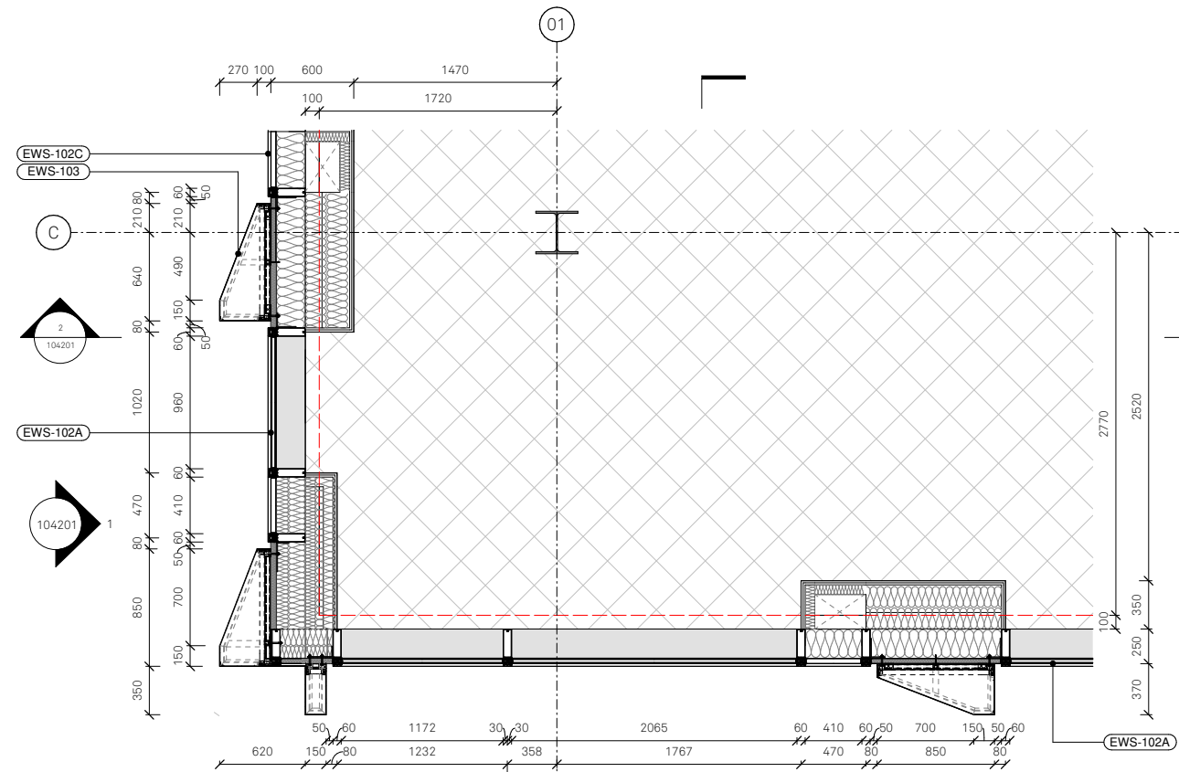
Level 04 - Plan 1 : 25
