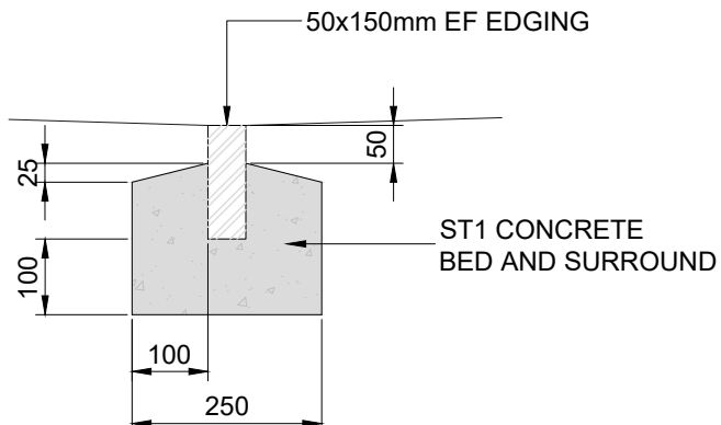
EK - FLAT TOP EDGING
