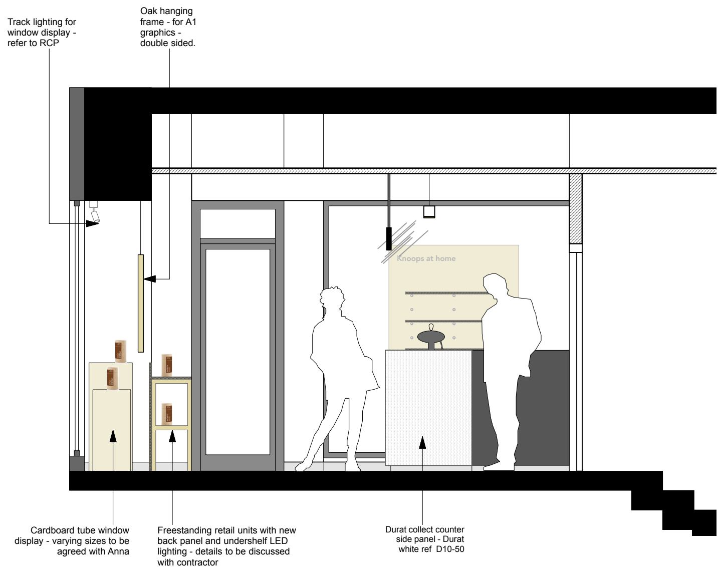
ELEVATION HH
