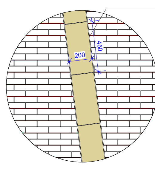
P2 Clay Pavers - Off Podium Scale: 1:20
