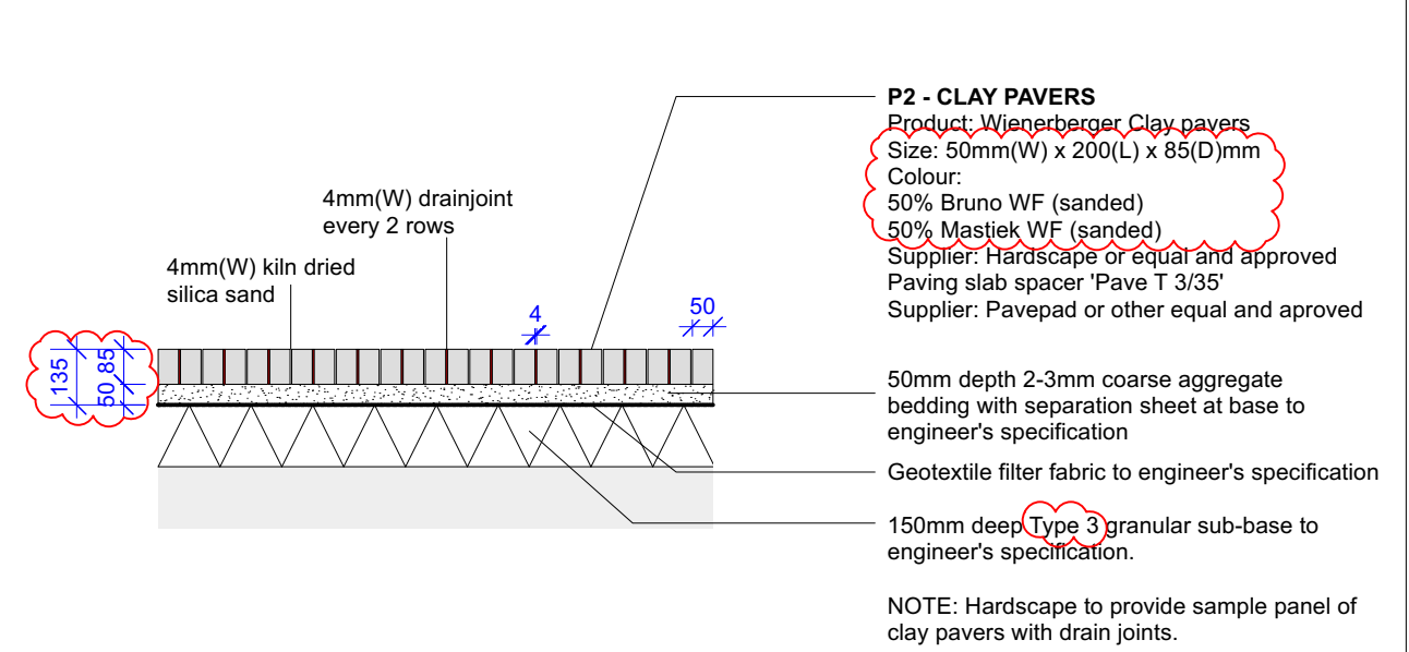
P2 Clay Pavers - Off Podium Scale: 1:20
