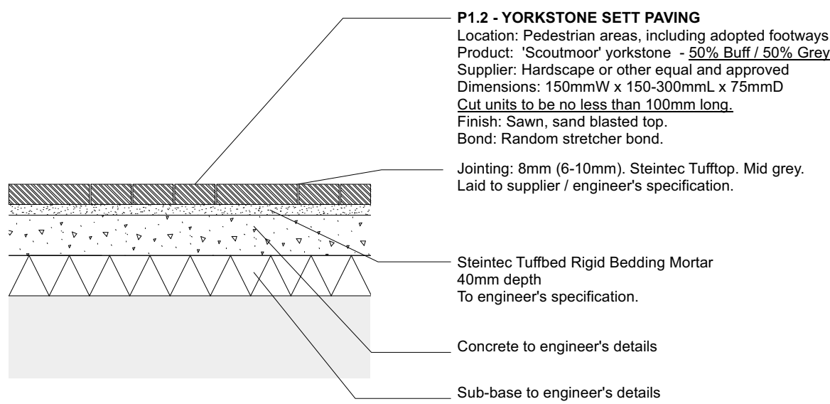
P1.2 Yorkstone Setts - to arrival spaces Scale: 1:20
