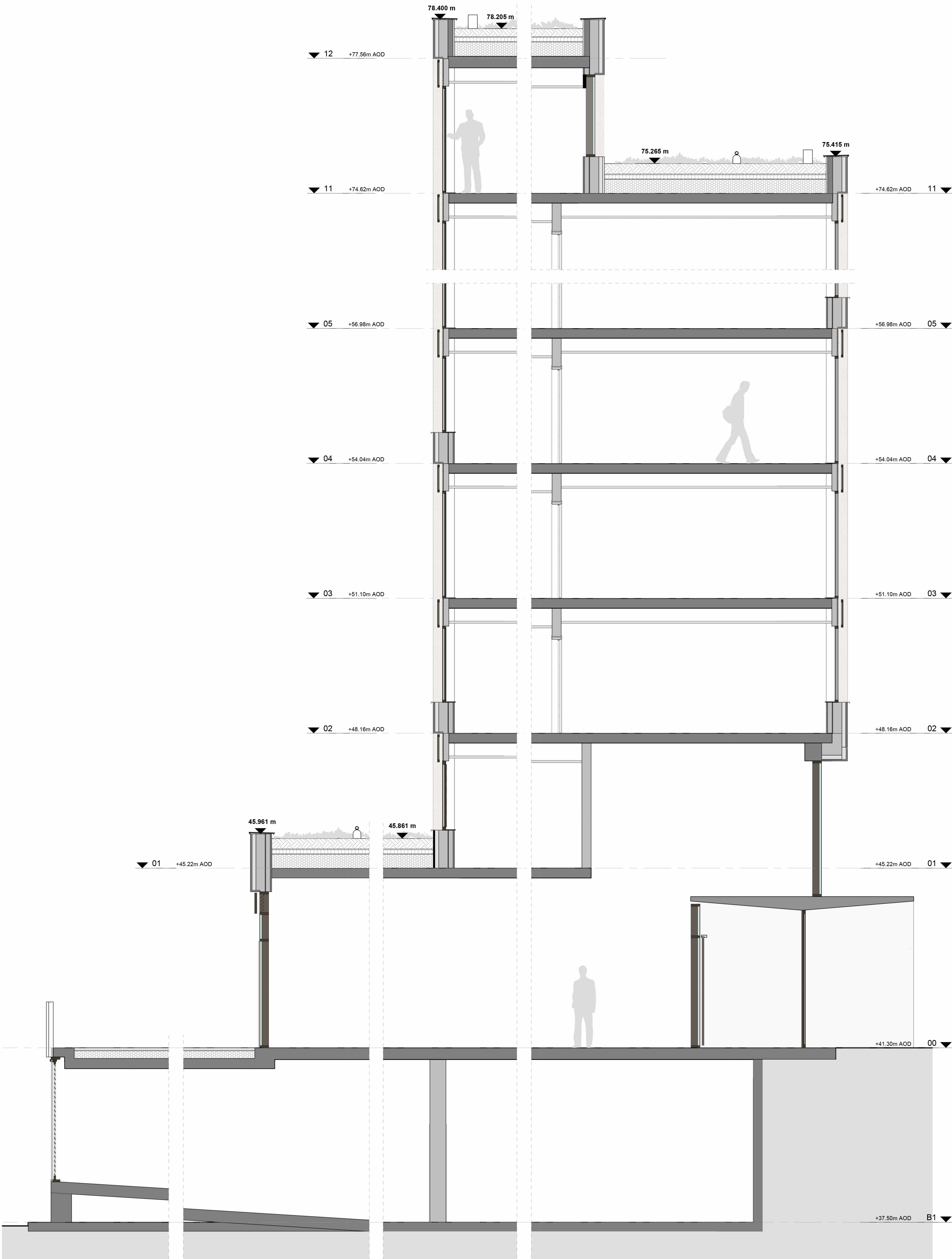
1 Strip Section 4 02403 1 : 50
