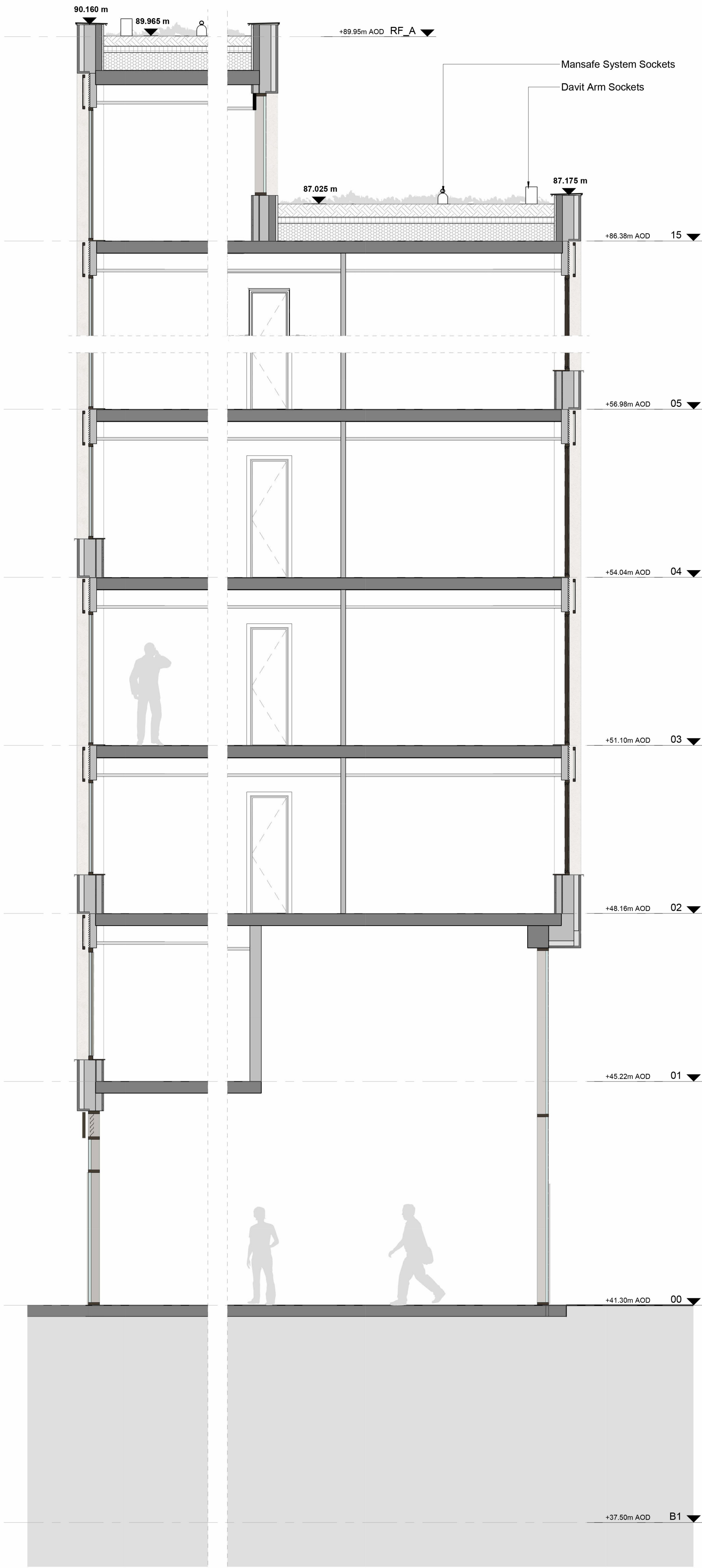
2 Strip Section 5 02403 1 : 50
