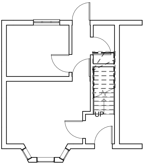
1 GF- Existing 1 : 100
