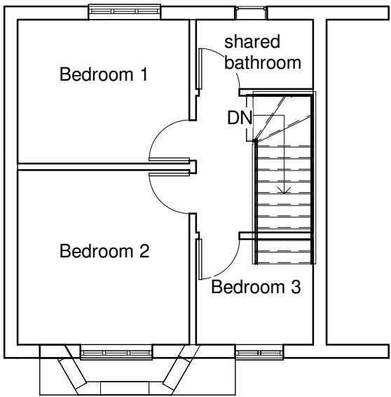
3 FF- Existing 1 : 100
