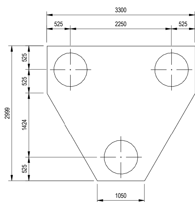
SCALE: 1 : 50
