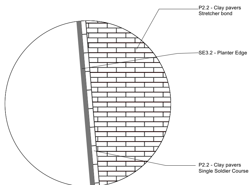
5 Detail Area 5 Scale: 1:25
