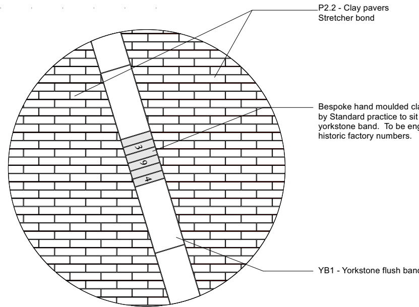
6 Detail Area 6 Scale: 1:25
