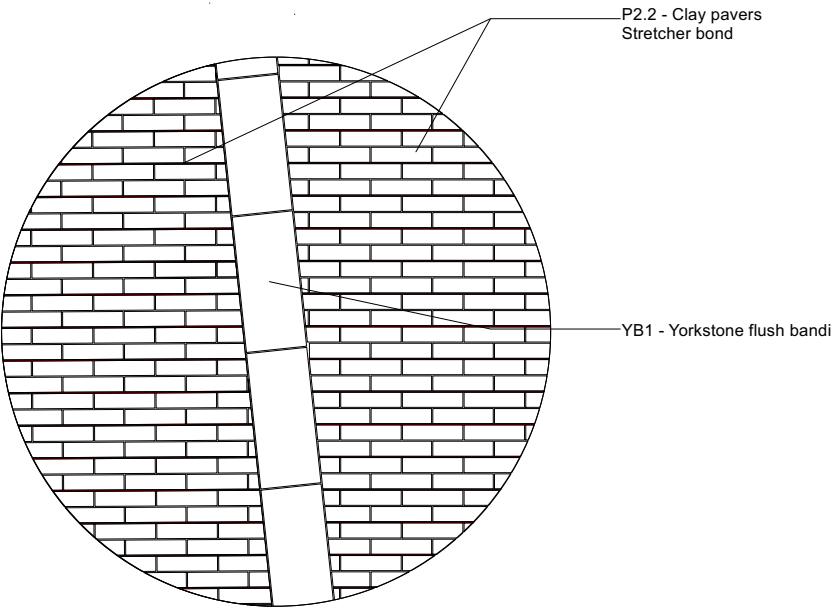
3 Detail Area 3 Scale: 1:25
