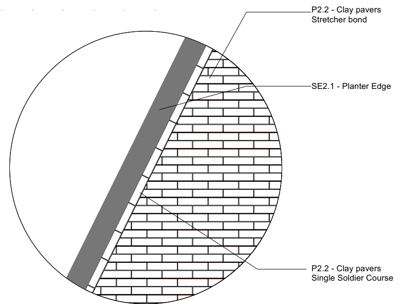
4 Detail Area 4 Scale: 1:25
