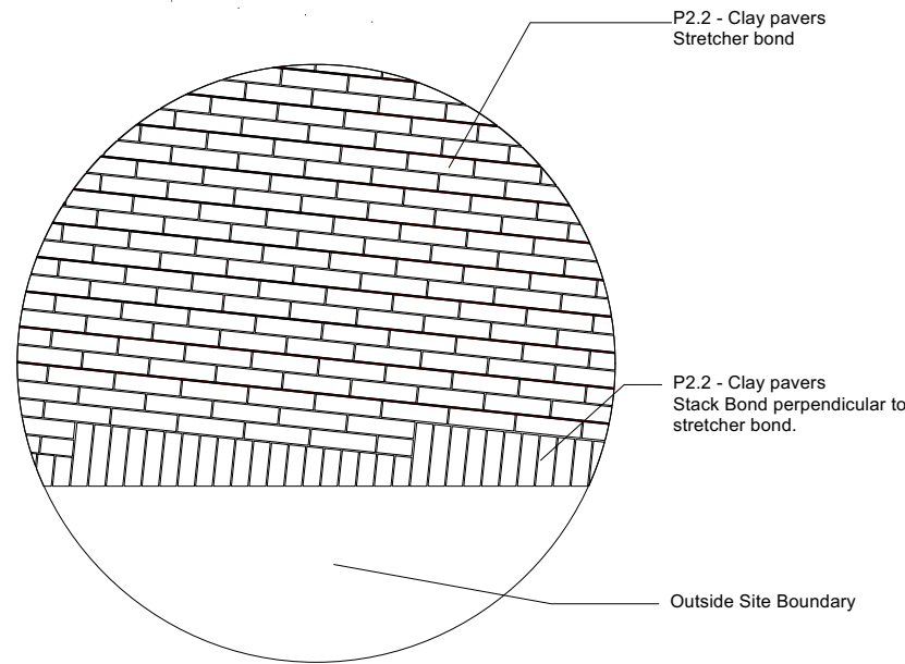
1 Detail Area 1 Scale: 1:25
