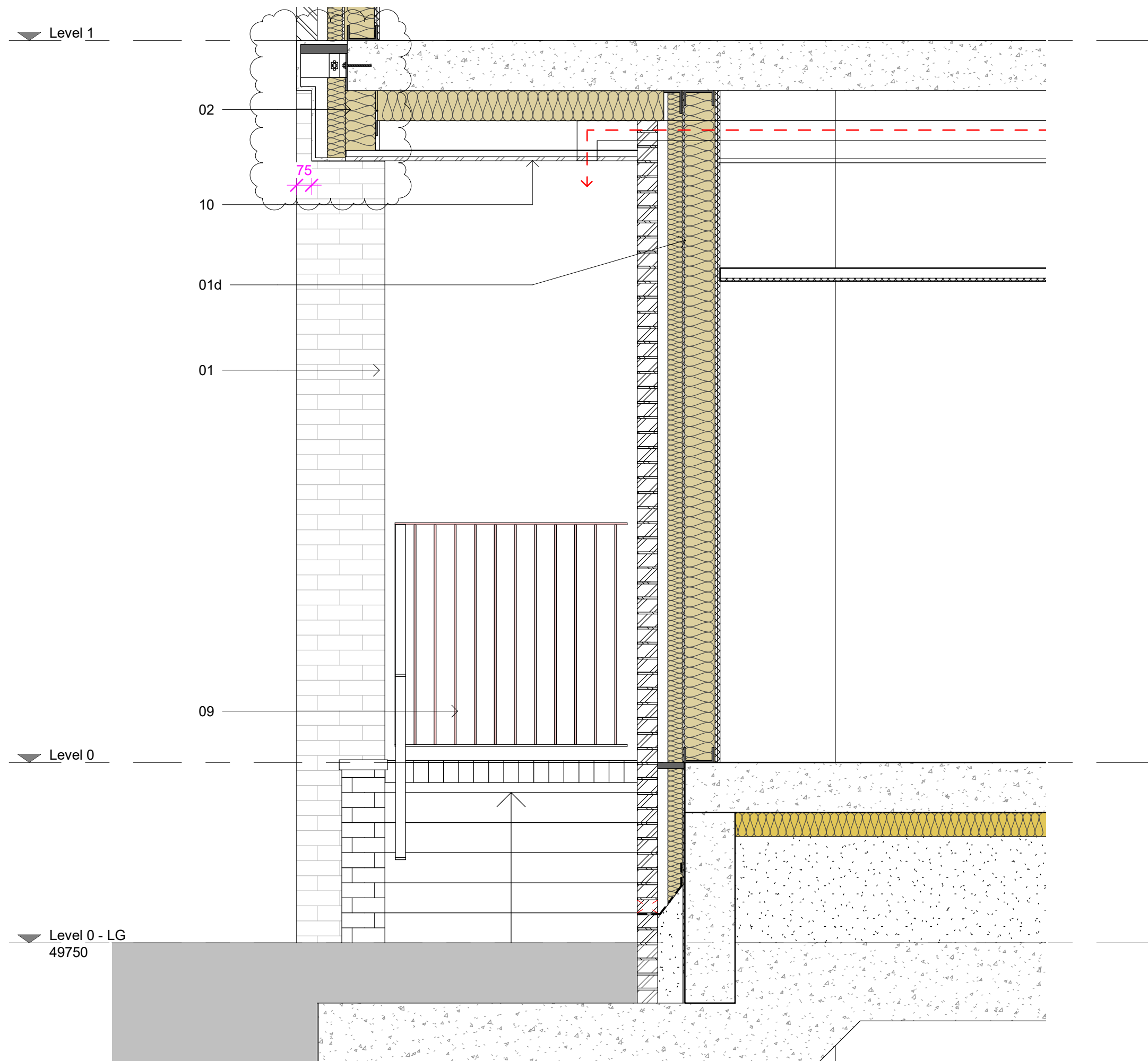
Section 01 1 : 20
