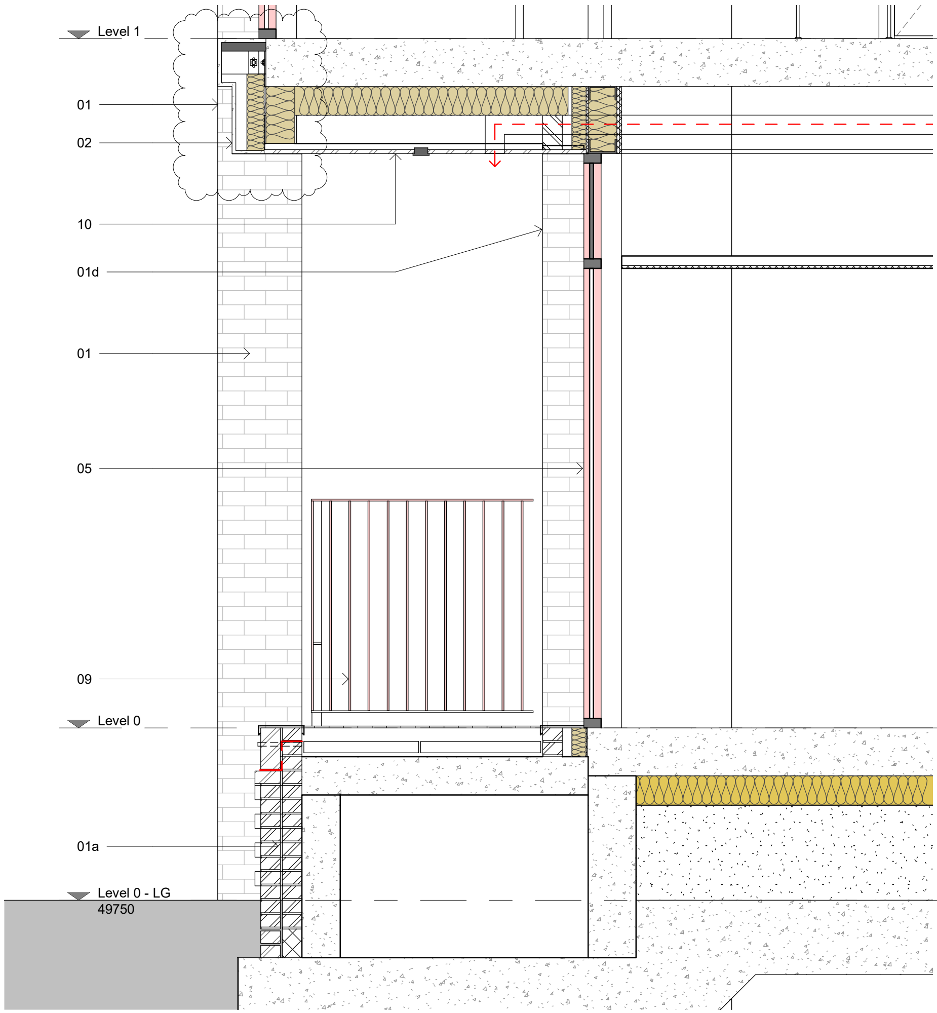
Section 2 1 : 20
