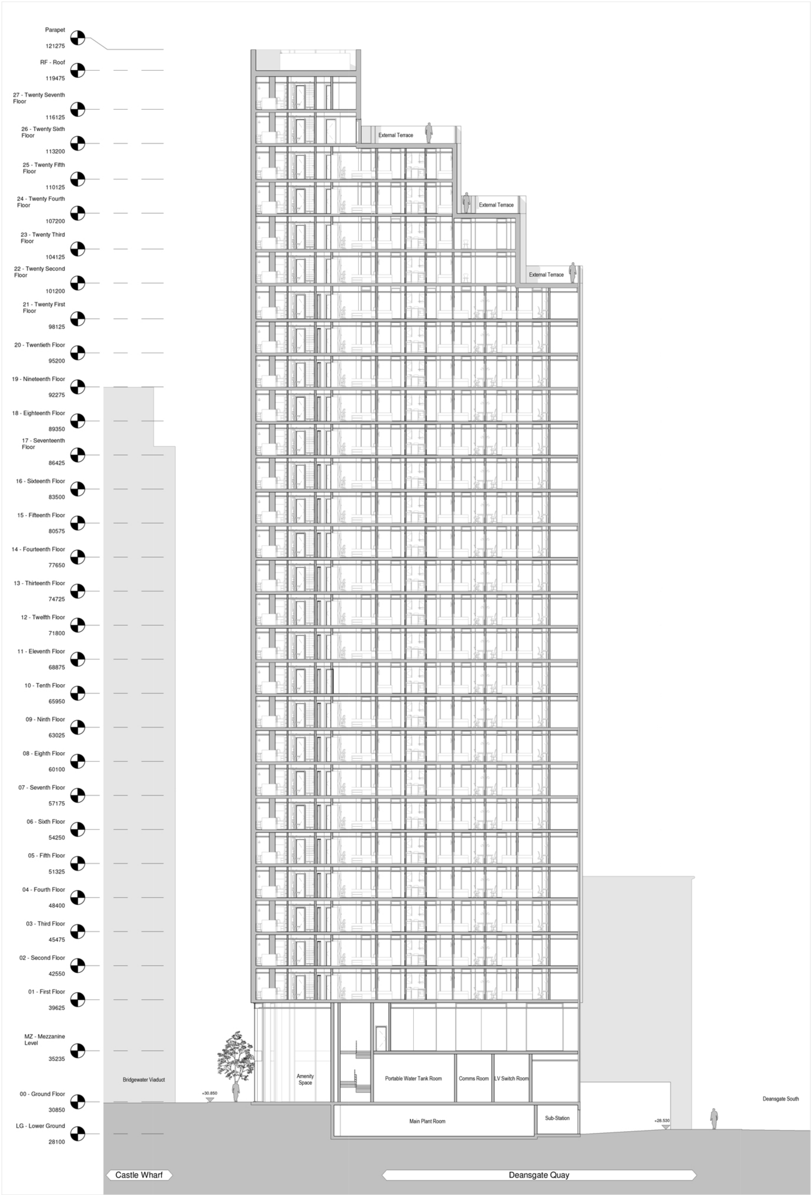
01 Section C-C 1 : 200
