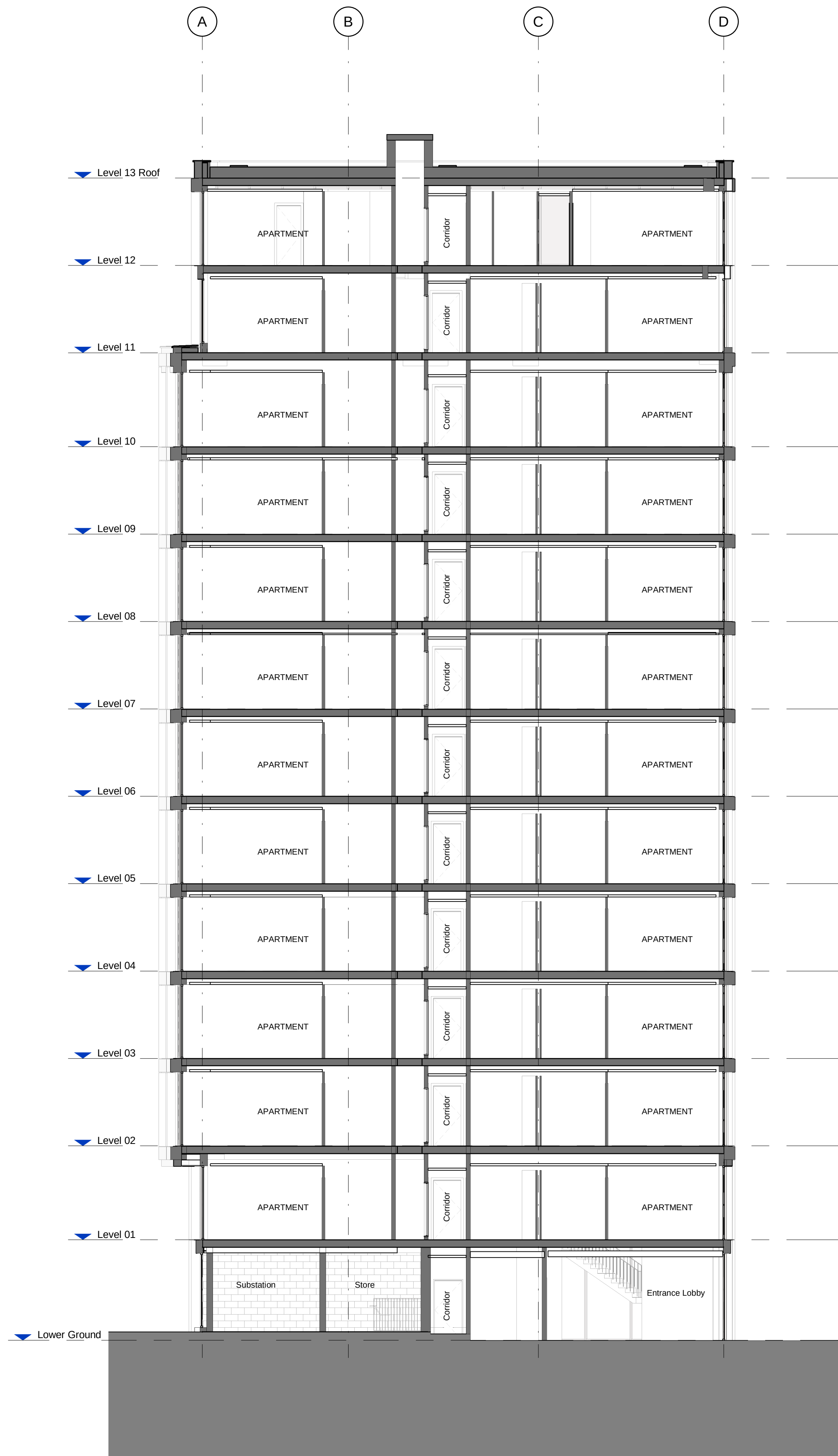
Section BB 1 : 100
