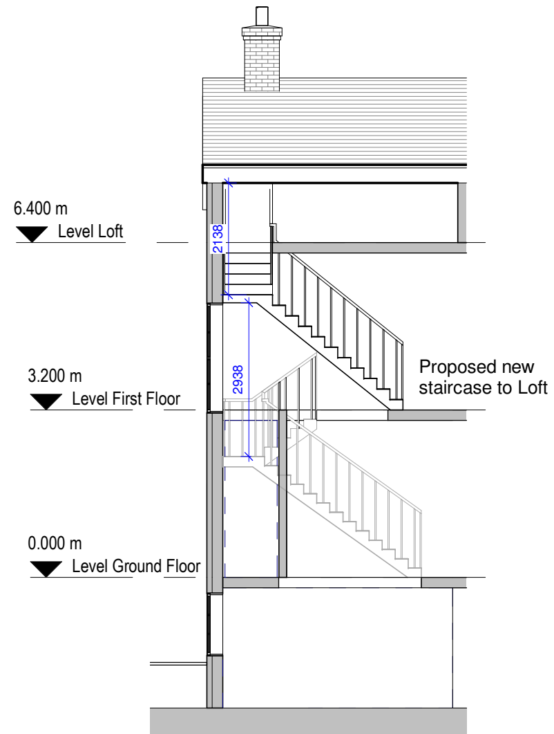
2 Section B-B 1 : 100
