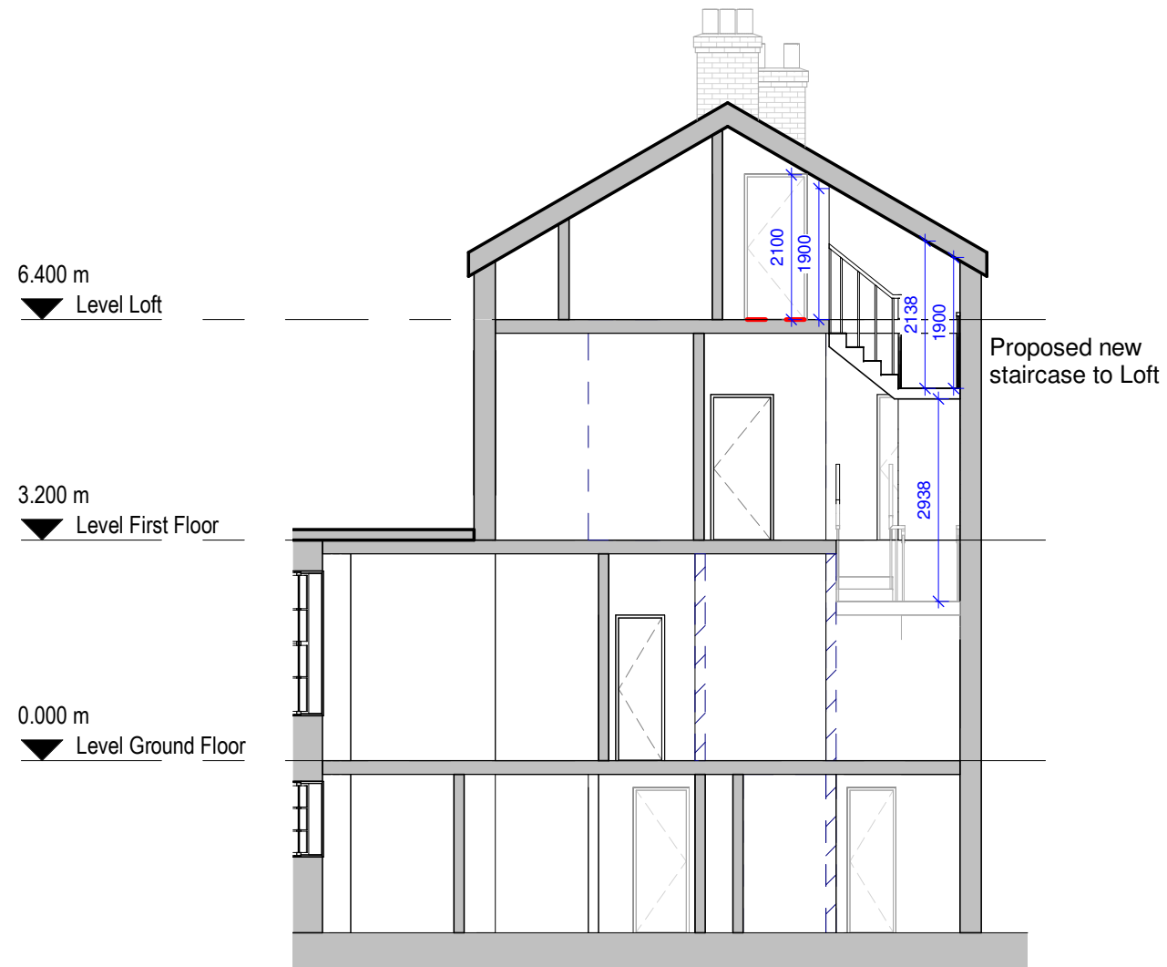
1 Section A-A 1 : 100
