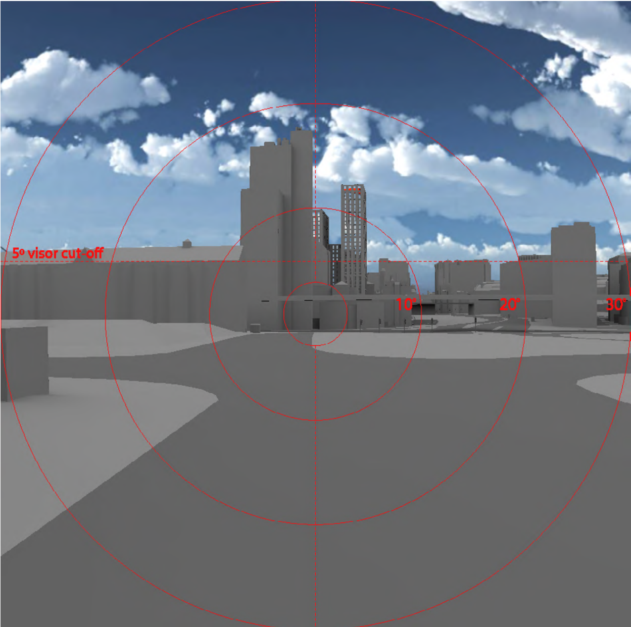
Fig. 69: Solar reflections
