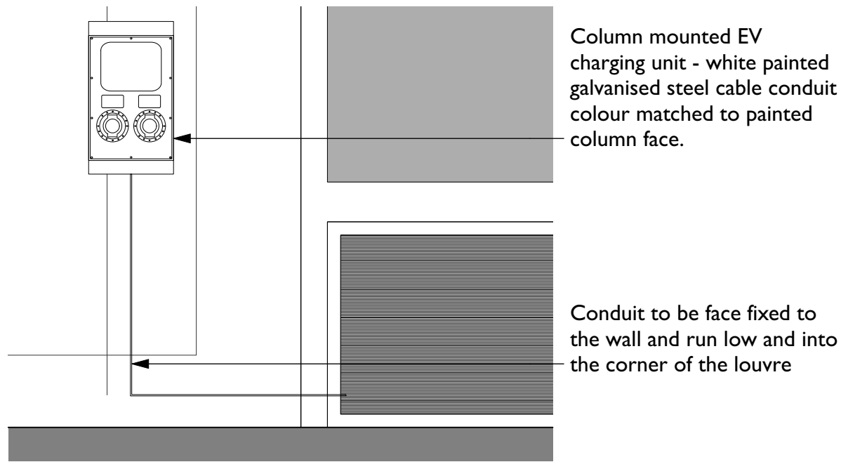
2 Rolec EV Charging Point Scale: 1:20
