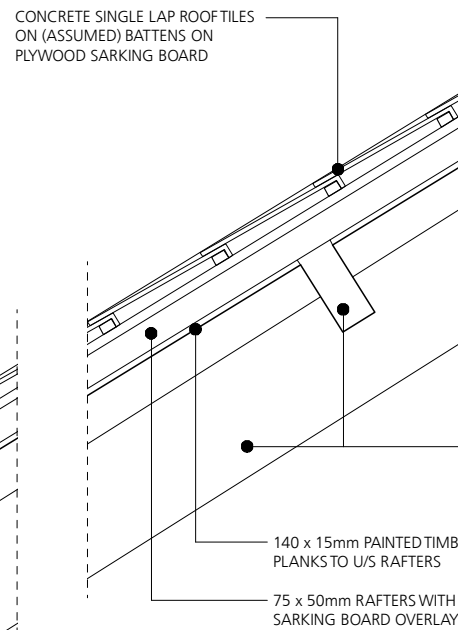
DETAIL E3
