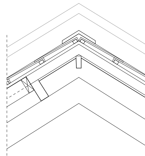
DETAIL E4
