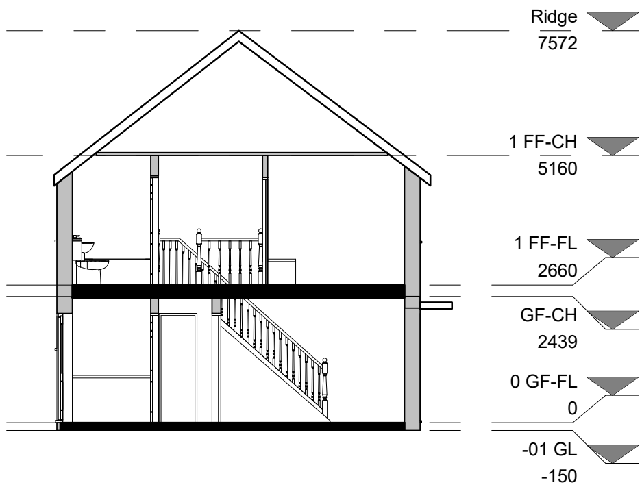
Section A-A 1 : 100
