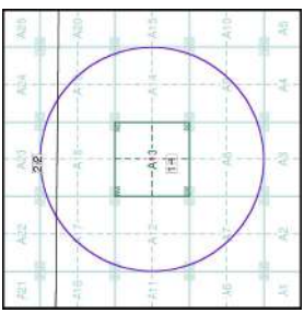
Superficial Geology Map - Slice A
