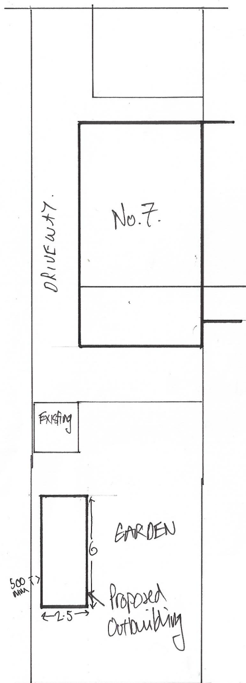
Site Plan 1:200
