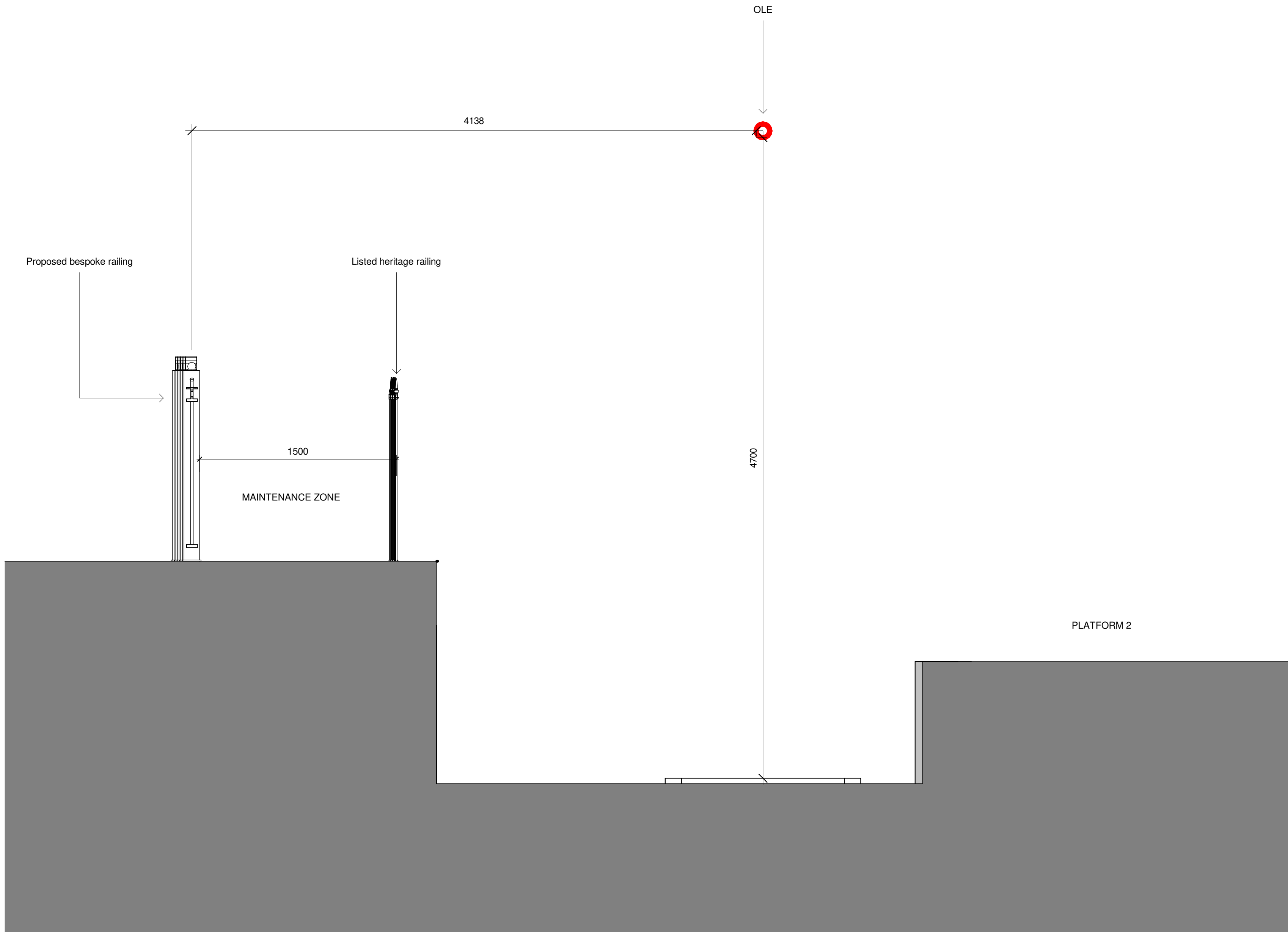
2 OLE Clearance 1 : 20
